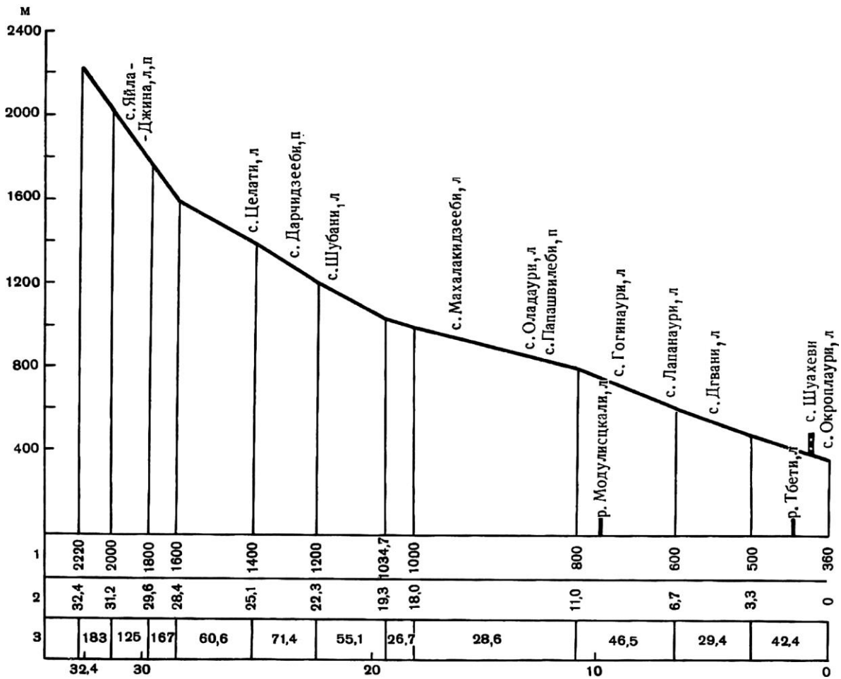
Рис. 4.1.49. Схематический продольный профиль р. Чирухис-Цкали
