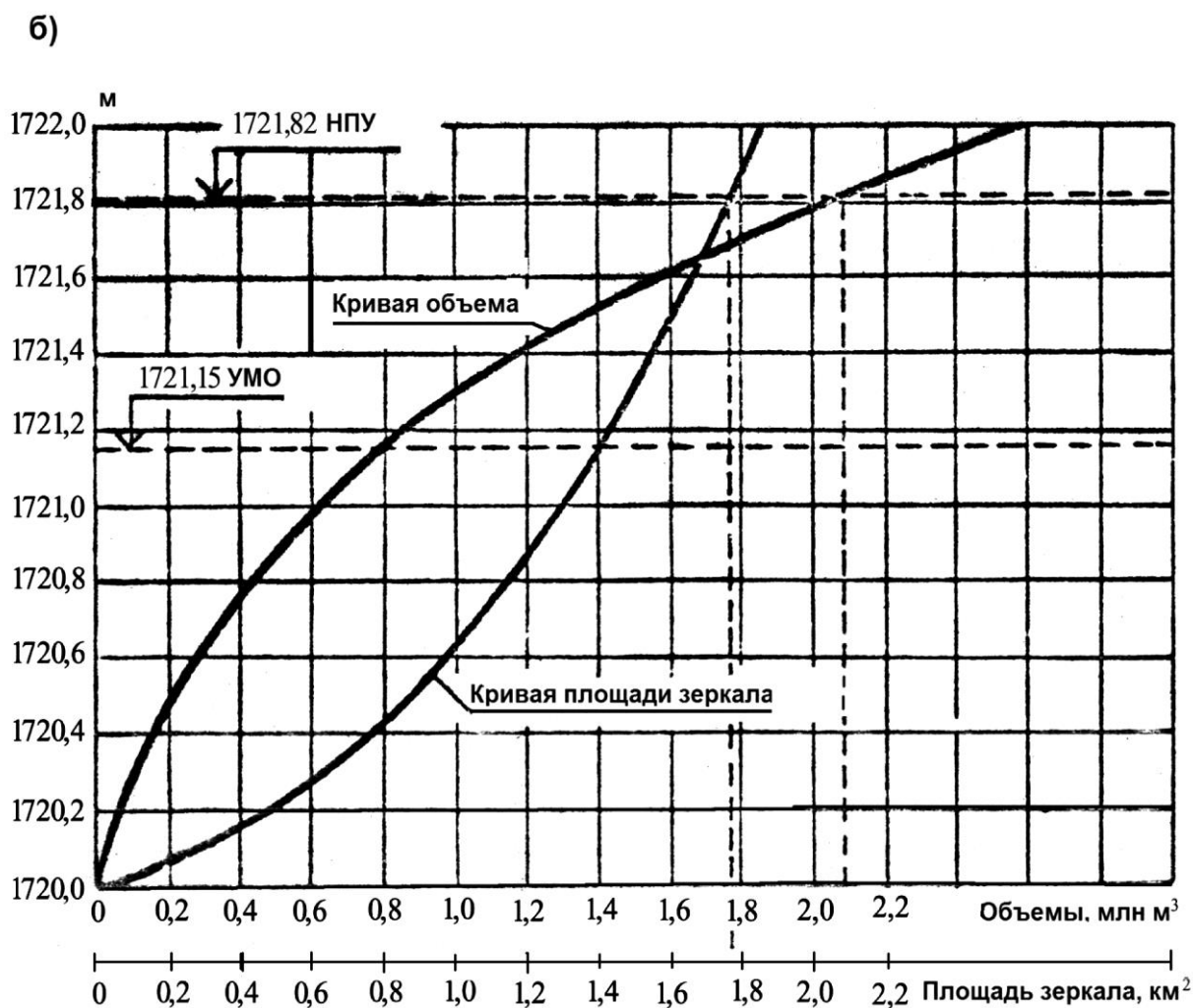
Рис. 4.2.21. Зресское водохранилище а) схема водохранилищной системы; б) график площади зеркала и объема водохранилища
