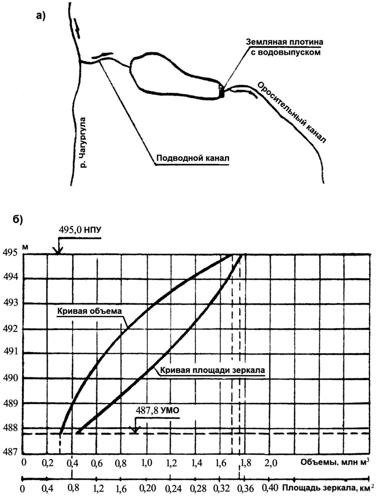
Рис. 4.2.14. Чальское водохранилище: а) схема водохранилищной системы; б) график площади зеркала и объема водохранилища
