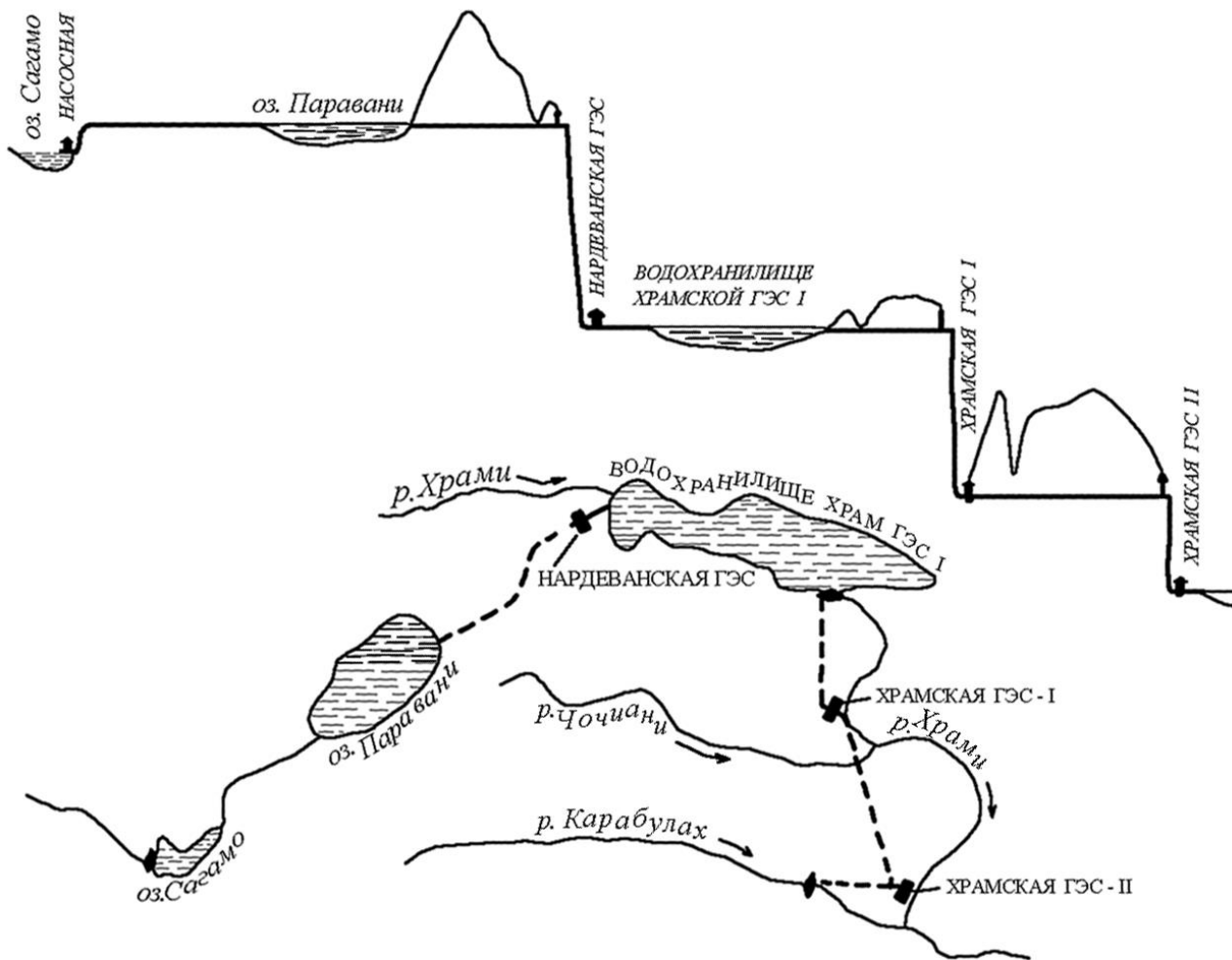
Рис. 4.2.4. Схема использования р. Храми
