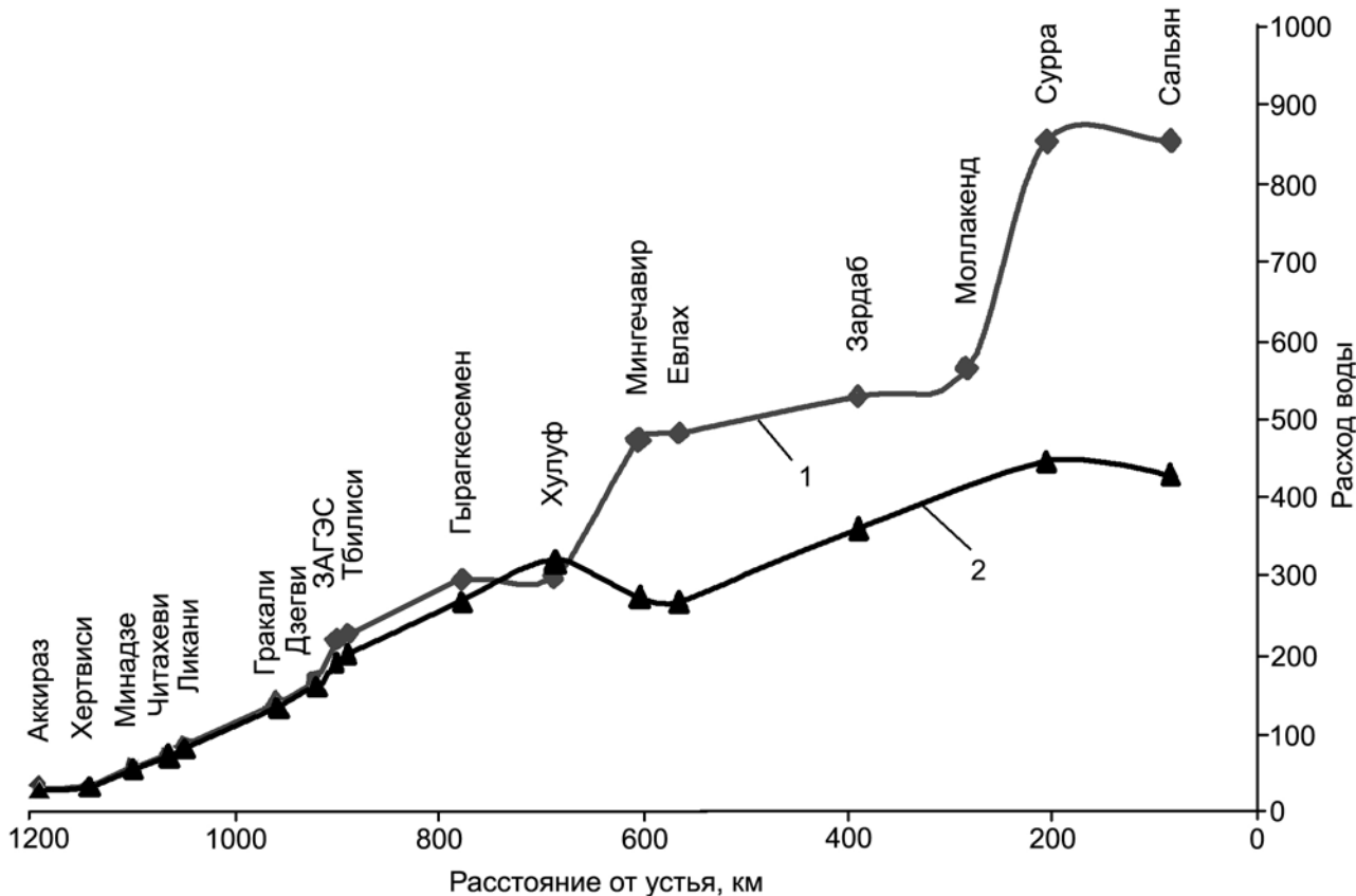
Рис. 7.2. Естественная и антропогенная трансформация годового стока реки Куры по ее длине: 1 – условно-естественный сток; 2-наблюдаемый сток (1991-2012 гг.).
