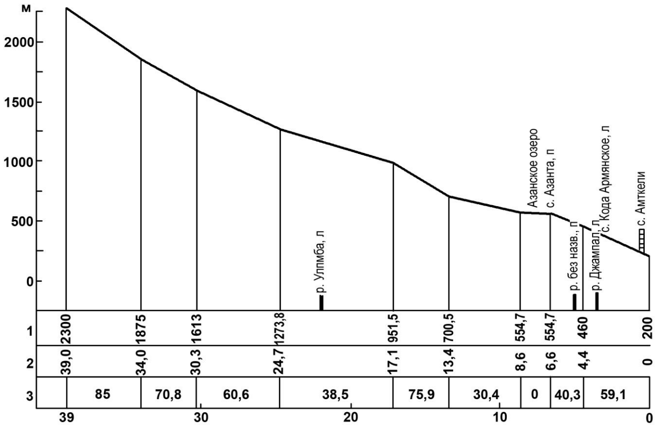
Рис. 4.1.21. Продольный профиль р. Амткели
