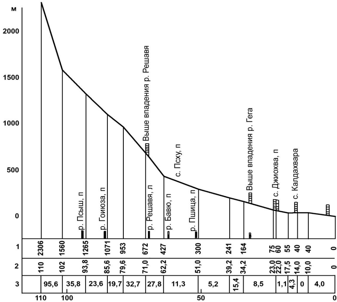
Рис. 4.1.13. Продольный профиль р. Бзыбь
