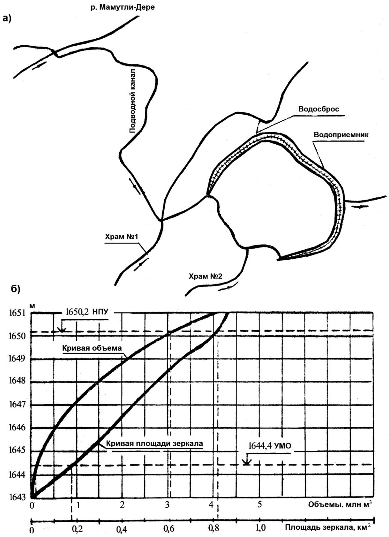
Рис. 4.2.20. Мтис-Дзирское водохранилище: а) схема водохранилищной системы; б) график площади зеркала и объема водохранилища
