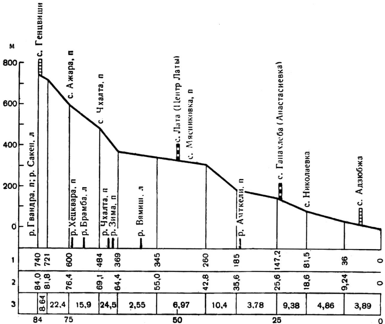
Рис. 4.1.19. Продольный профиль р. Кодори
