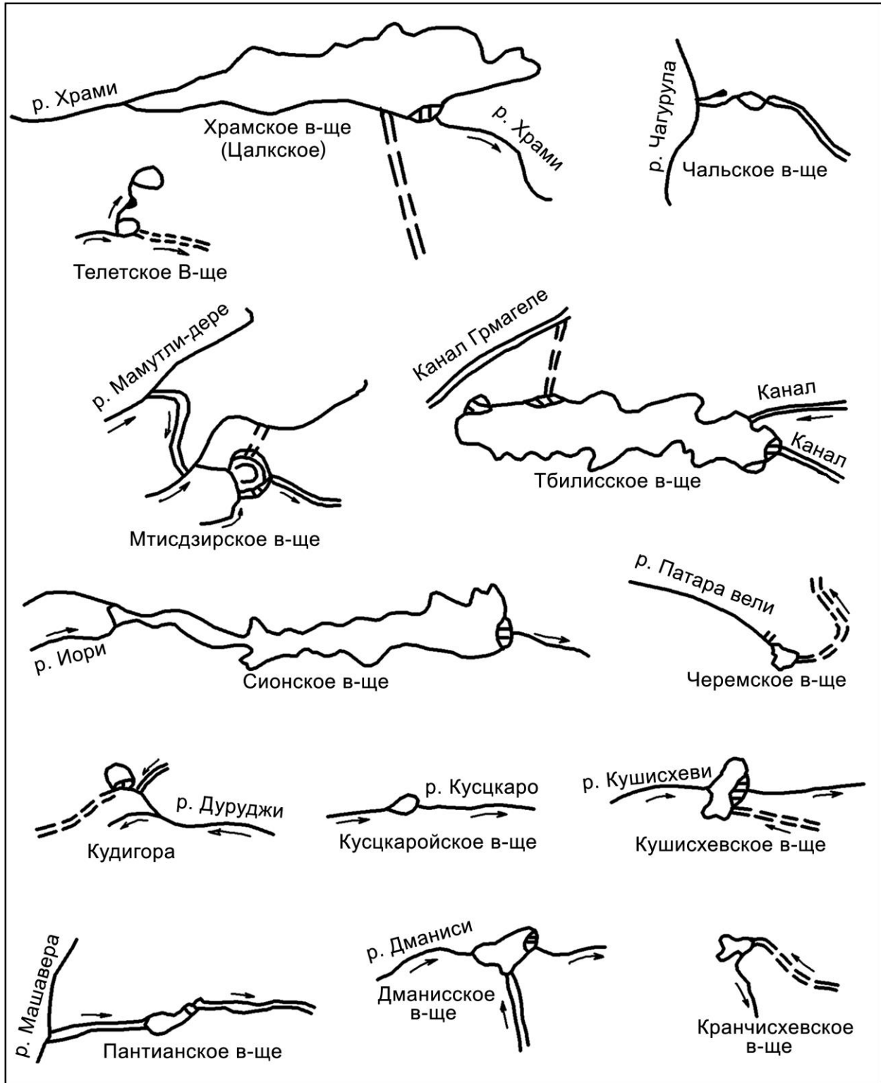
Рис. 4.2.3-а. Формы водохранилищ Восточной Грузии (в соотносительном масштабе) (— — реки; — — — — — каналы; == == == — водотоки, водосбросы, водоприемники и т.д.)
