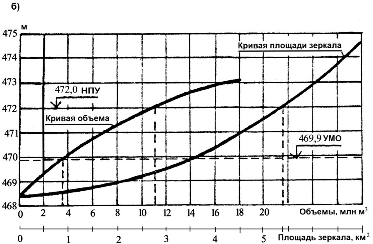
Рис. 4.2.22. Кумисское водохранилище: а) схема водохранилищной системы; б) график площади зеркала и объема водохранилища
