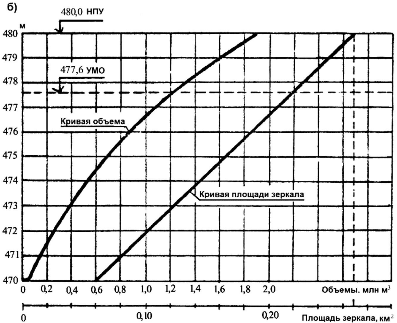
Рис. 4.2.13. Кранчис-Хевское водохранилище (не функционирует): а) схема водохранилищной системы; б) график площади зеркала и объема водохранилища
