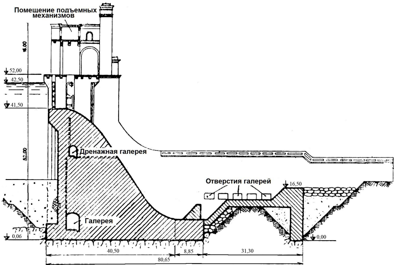
Рис. 4.2.47. Головной узел Гуматского водохранилища: а) план; б) поперечный профиль бетонной плотины
