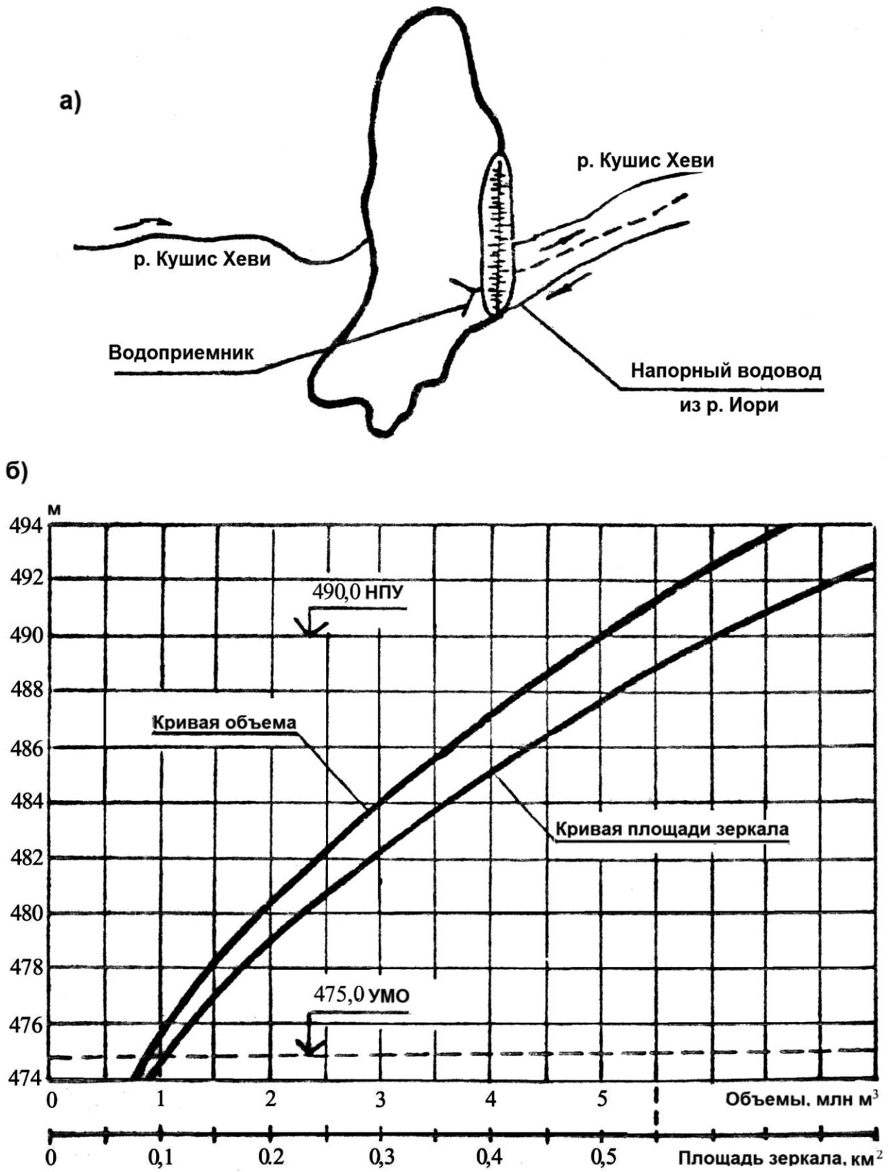
Рис. 4.2.17. Кушис-Хевское водохранилище: а) схема водохранилищной системы; б) график площади зеркала и объема водохранилища
