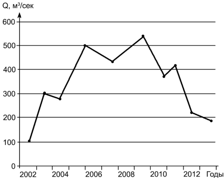
Рис. 7.1. Гидрограф среднегодовых расходов реки Чорохи
