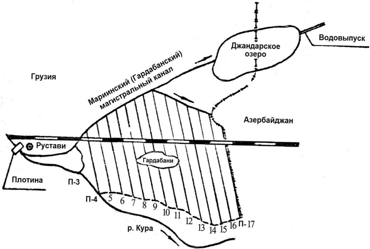
Рис. 4.2.26. Схема Джандарской водохранилищной системы
