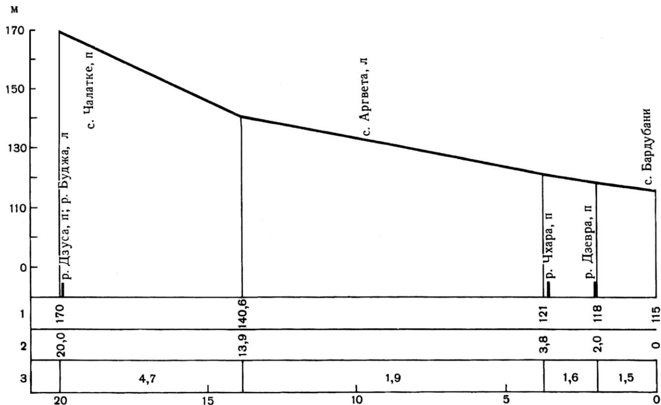
Рис. 4.1.37. Схематический продольный профиль р. Чолабури
