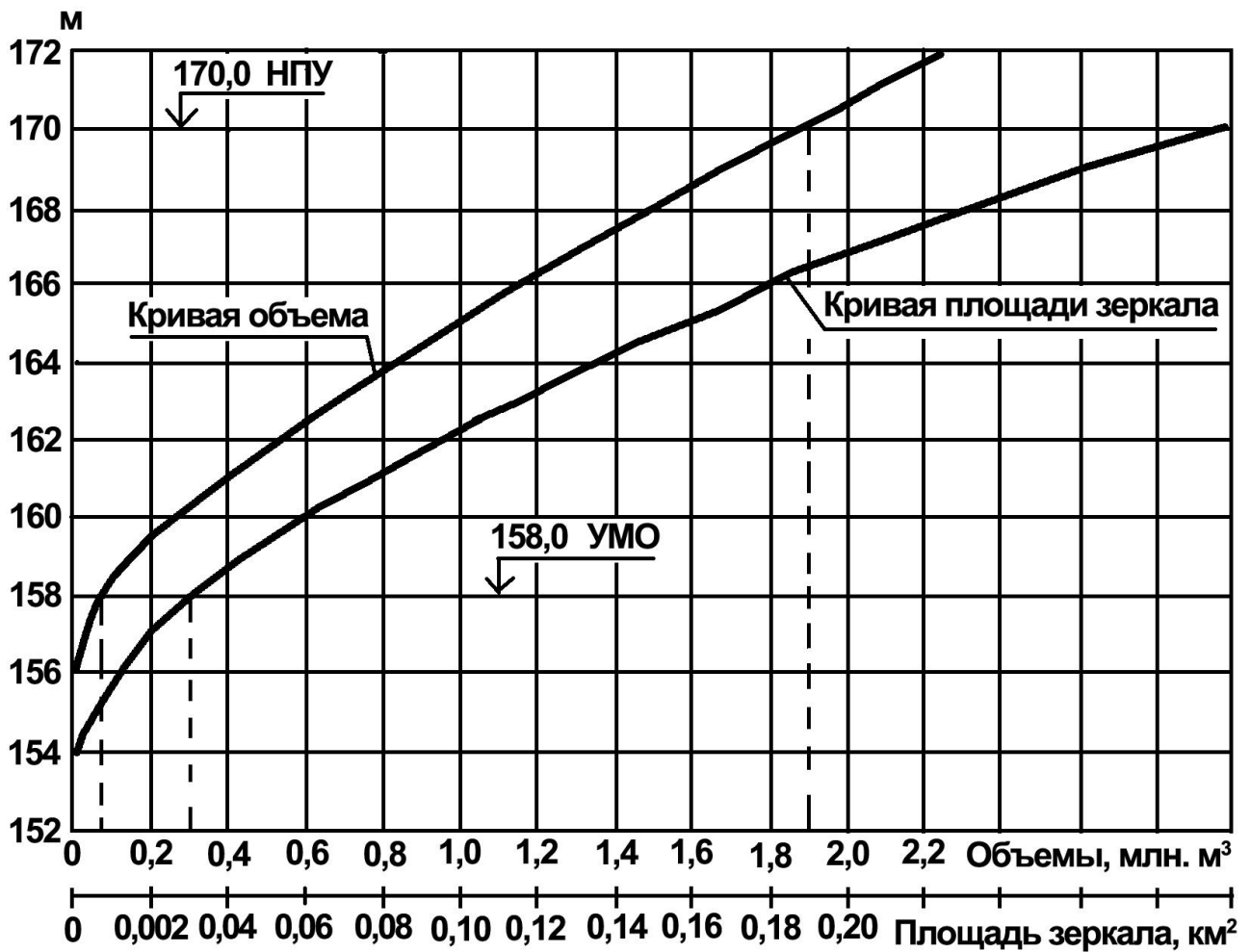
Рис. 4.2.37. Кухское водохранилище а) схема водохранилищной системы; б) график площади зеркала и объема водохранилища
