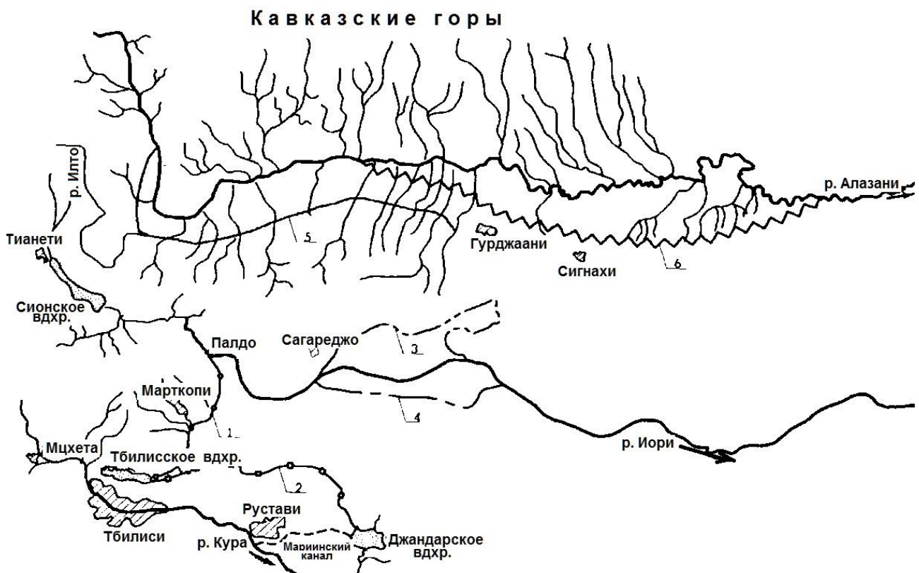
Рис. 4.2.55. Схема Самгорской и Алазанской оросительных систем:
