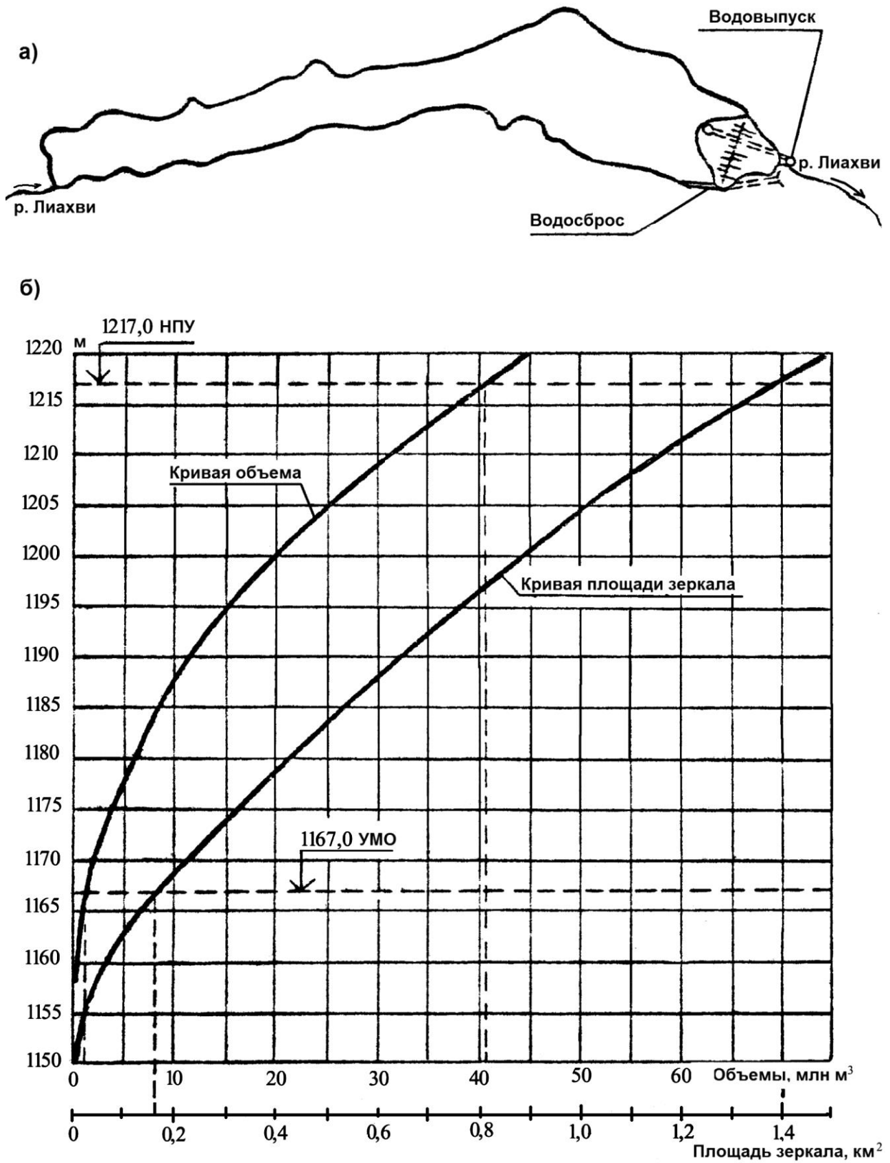
Рис. 4.2.9. Зонкарское (Патара Лиавхское) водохранилище: а) схема водохранилищной системы; б) график площади зеркала и объема водохранилища
