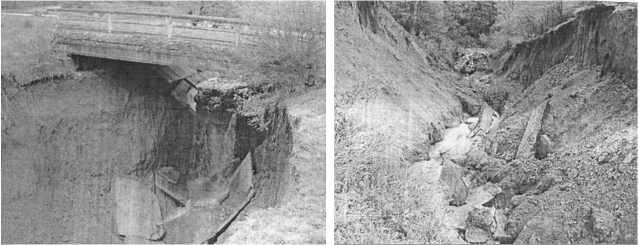
Фото 4.2.3. Авария на водосбросе Черемского водохранилища
