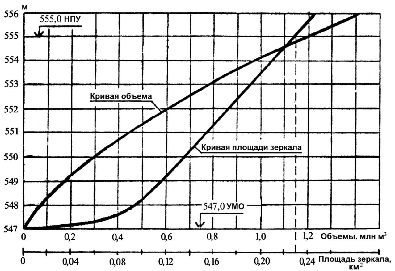
Рис. 4.2.12. Марабдинское водохранилище: а) схема водохранилищной системы; б) график площади зеркала и объема водохранилища
