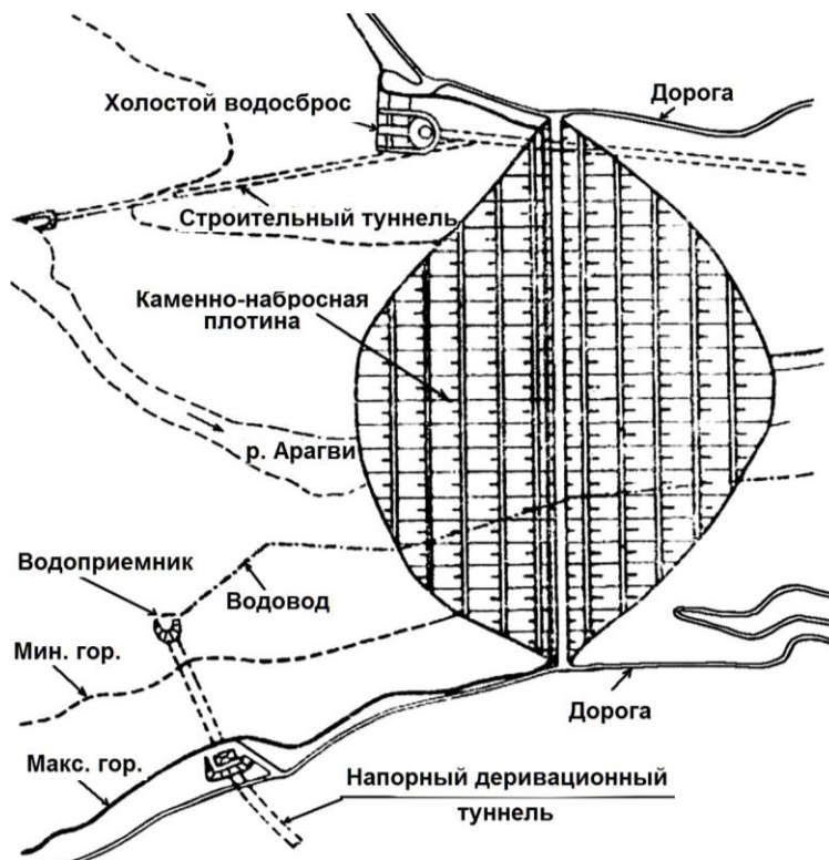
Рис. 4.2.46. Головной узел Жинвальского водохранилища
