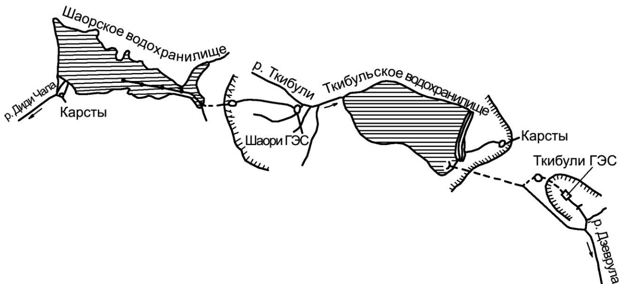
Рис. 4.2.33. Схема Шаори-Ткибульского каскада водохранилищ
