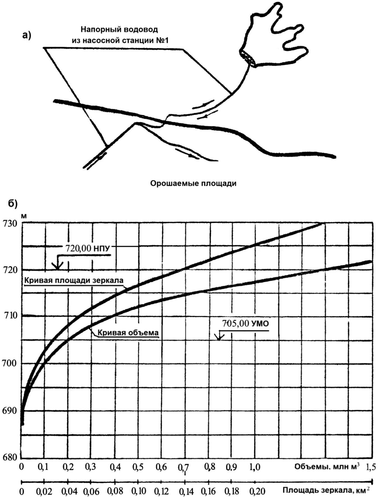
Рис. 4.2.16. Телет-Цкальское водохранилище (не функционирует): а) схема водохранилищной системы; б) график площади зеркала и объема водохранилища
