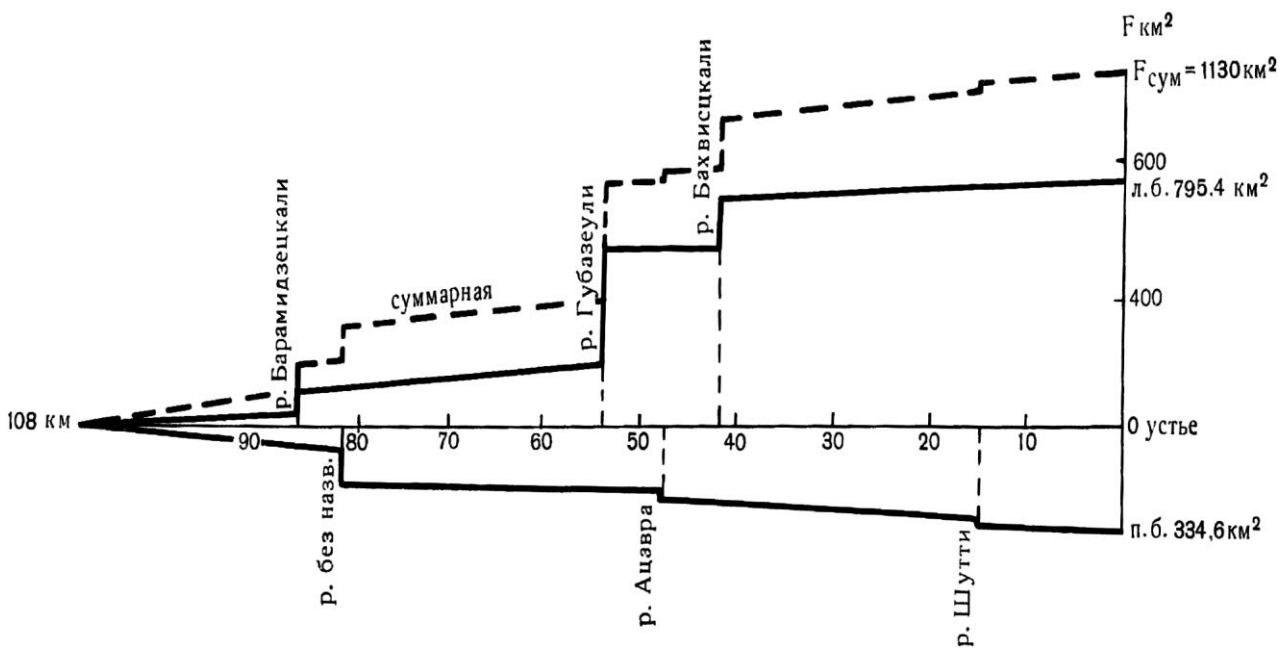
Рис. 4.1.44. График роста площади бассейна р. Супса
