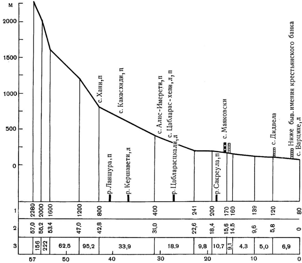
Рис. 4.1.39. Схематический продольный профиль р. Ханис-Цкали
