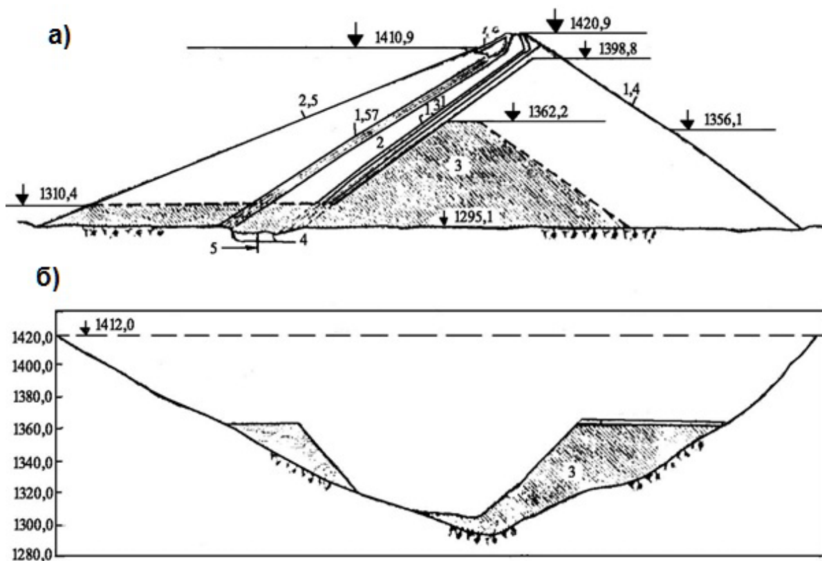
Рис. 1.9.1. Авария на плотине Хел-Хол из-за перелива воды через гребень плотины: а) поперечный профиль : 1 – насыпь; 2 – экран из грунта; 3 – остатки плотины после наводнения; 4 – цементация; 5 – цементационная завеса.
