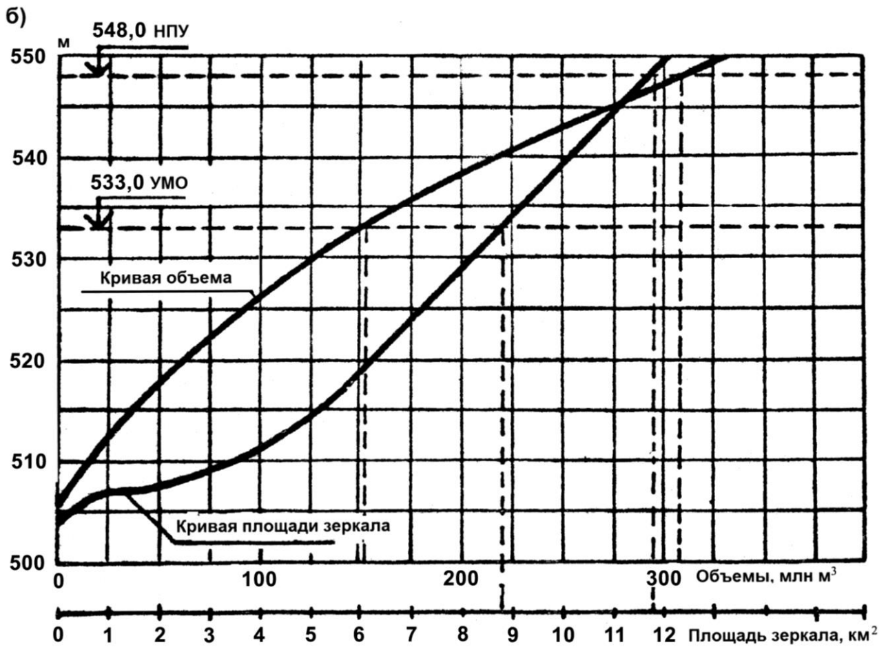
Рис. 4.2.6. Тбилисское водохранилище: а) схема водохранилищной системы; б) график площади зеркала и объема водохранилища
