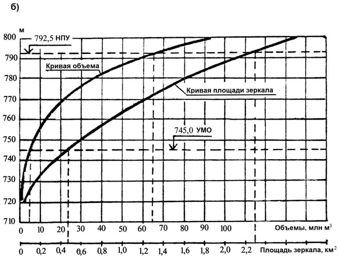
Рис. 4.2.10. Алгетское водохранилище: а) схема водохранилищной системы; б) график площади зеркала и объема водохранилища
