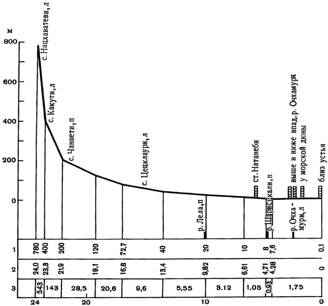
Рис. 4.1.47. Схематический продольный профиль р. Чолоки
