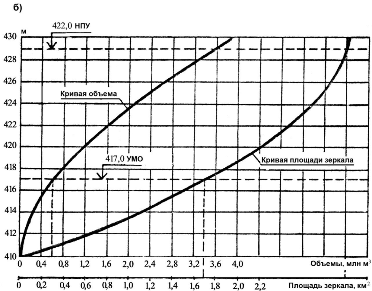
Рис. 4.2.19. Лапианское водохранилище: а) схема водохранилищной системы; б) график площади зеркала и объема водохранилища
