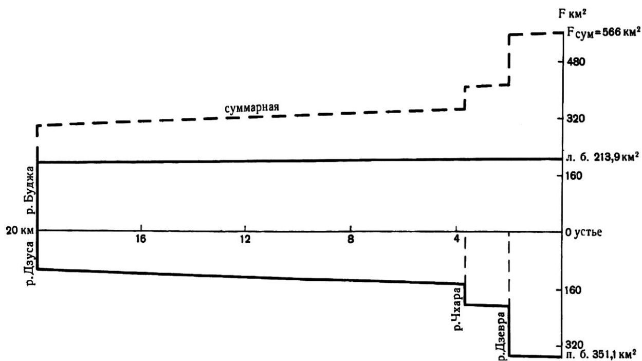
Рис. 4.1.37. Схематический продольный профиль р. Чолабури
