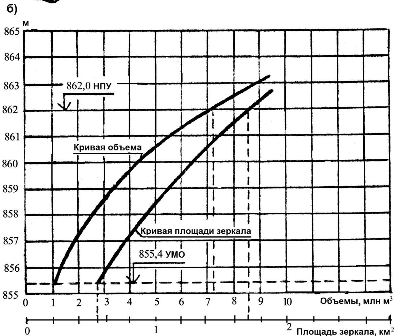
Рис. 4.2.23. Надарбазевское водохранилище а) схема водохранилищной системы; б) график площади зеркала и объема водохранилища
