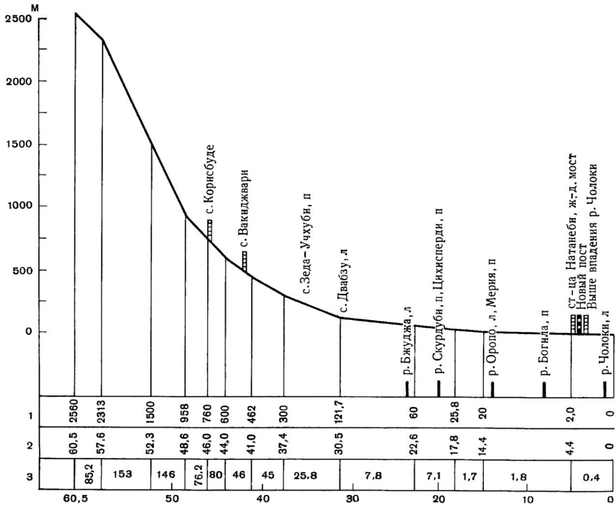
Рис. 4.1.45. Схематический продольный профиль р. Натанеби
