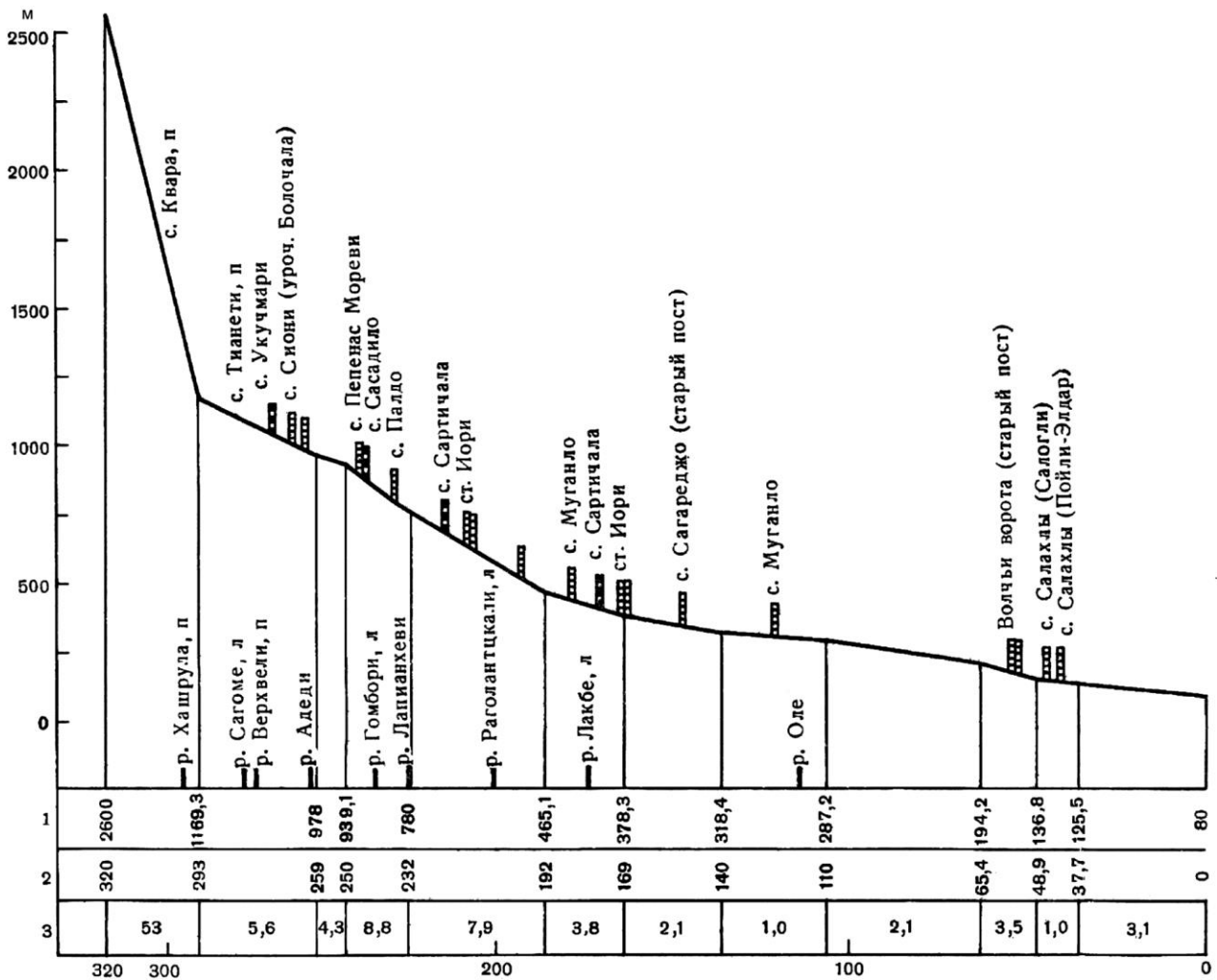
Рис. 4.1.8. Продольный профиль р. Иори
