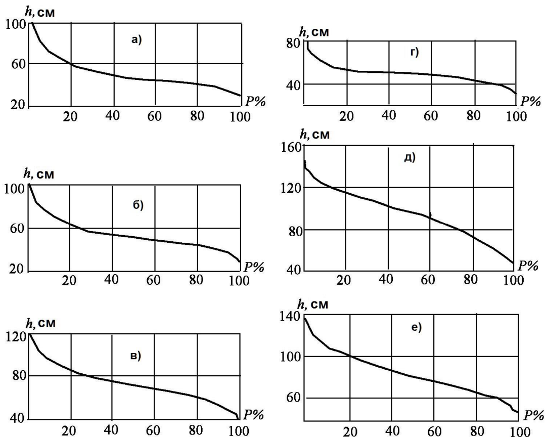
Рис. 4.2.38. Графики обеспеченности высот волн ( h ) на Гальском (а), Шаорском (б), Ткибульском (в), Сионском (г), Тбилисском (д), Храмском (е) водохранилищах
