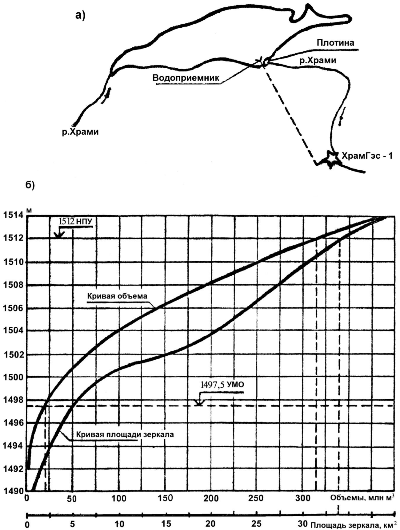
Рис. 4.2.7. Храмское водохранилище а) схема водохранилищной системы; б) график площади зеркала и объема водохранилища.
