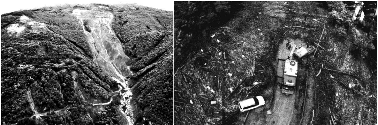
Фото 4.2.3. Авария на водосбросе Черемского водохранилища
