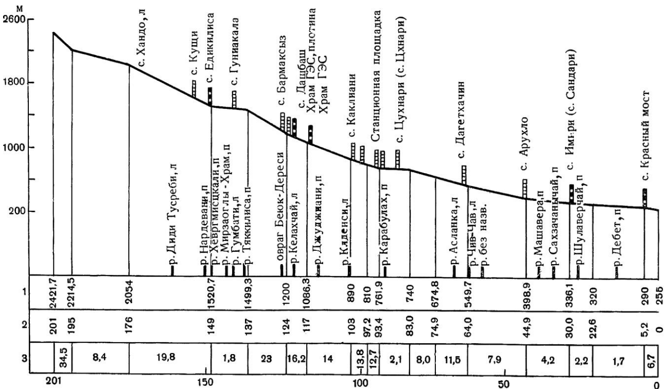
Рис. 4.1.5. Продольный профиль р. Храми
