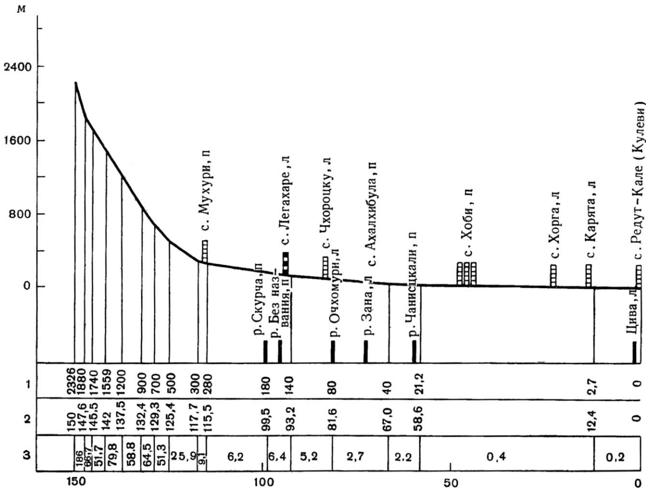
Рис. 4.1.29. Схематический продольный профиль р. Хоби
