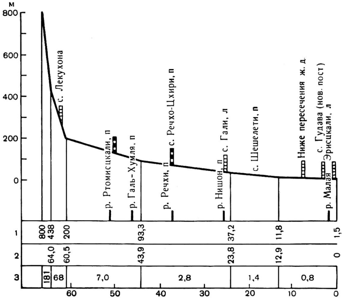
Рис. 4.1.25. Схематический продольный профиль р. Диди Эрис-Цкали
