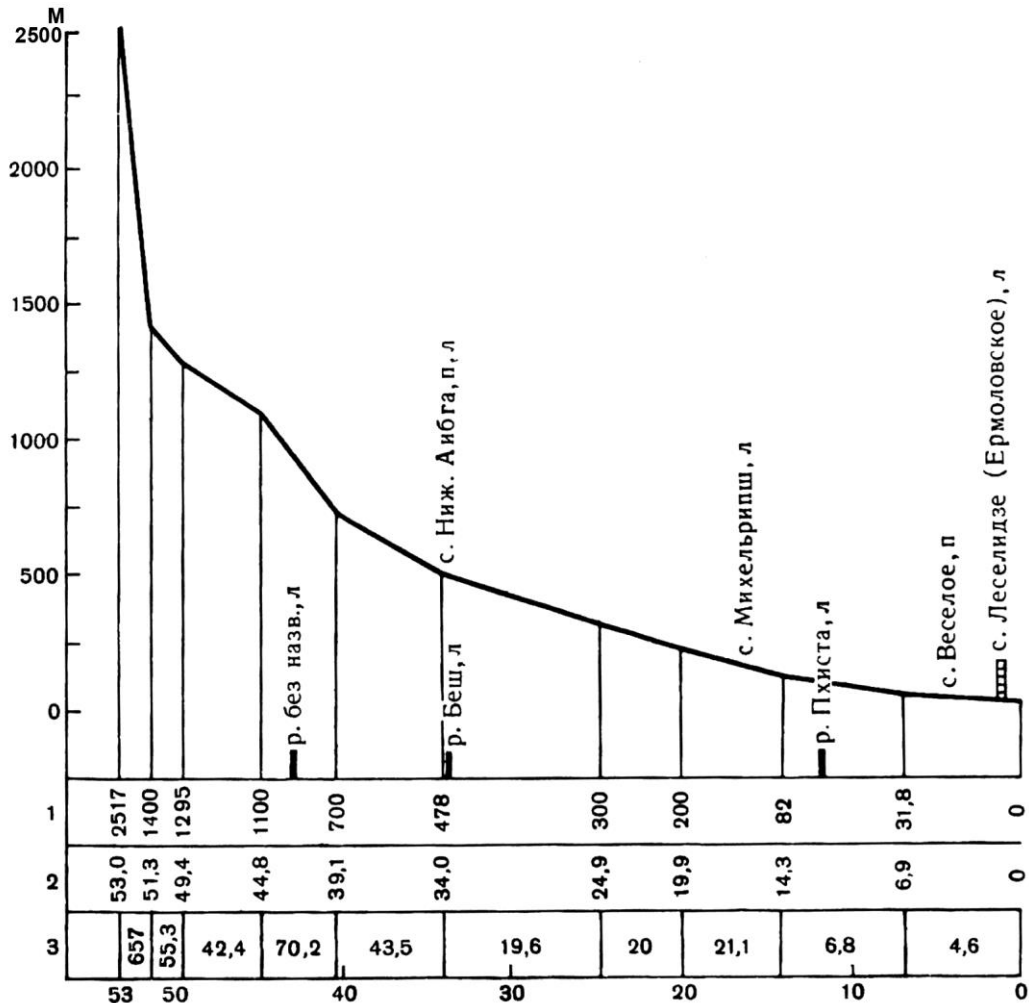
Рис. 4.1.11. Продольный профиль р. Псоу
