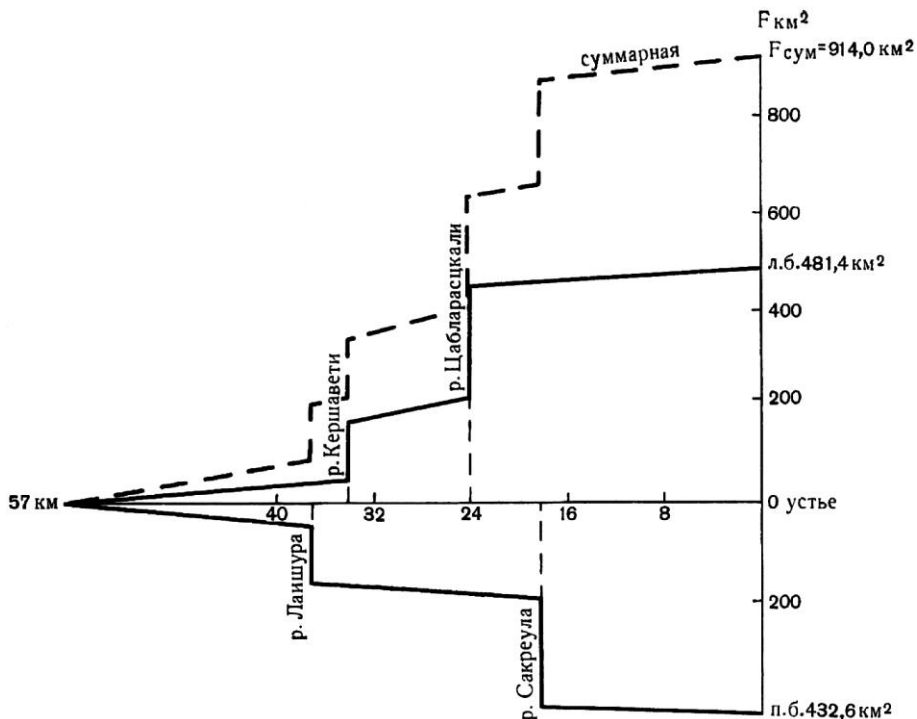
Рис. 4.1.40. График роста площади бассейна р. Ханис-Цкали
