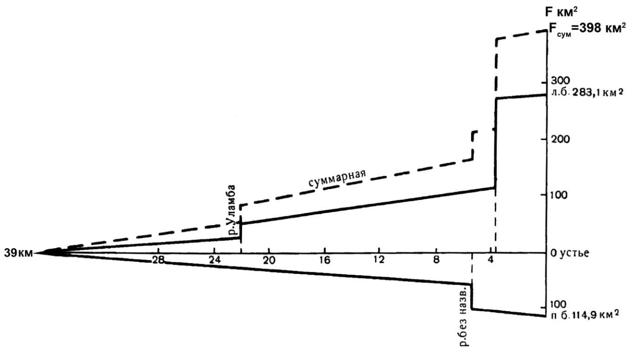
Рис. 4.1.22. График увеличения площади водосбора р. Амткели
