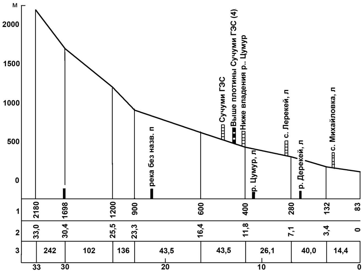
Рис. 4.1.17. Продольный профиль р. Восточной Гумисты
