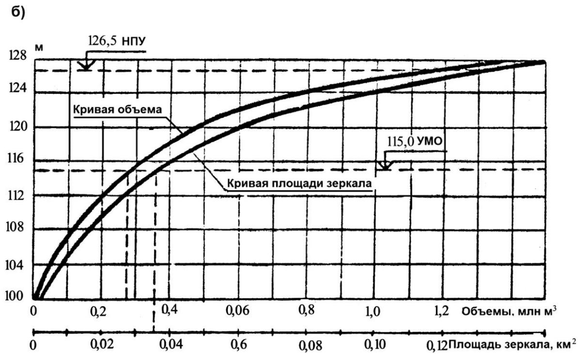
Рис. 4.2.11. Черемское водохранилище (не функционирует): а) схема водохранилищной системы; б) график площади зеркала и объема водохранилища
