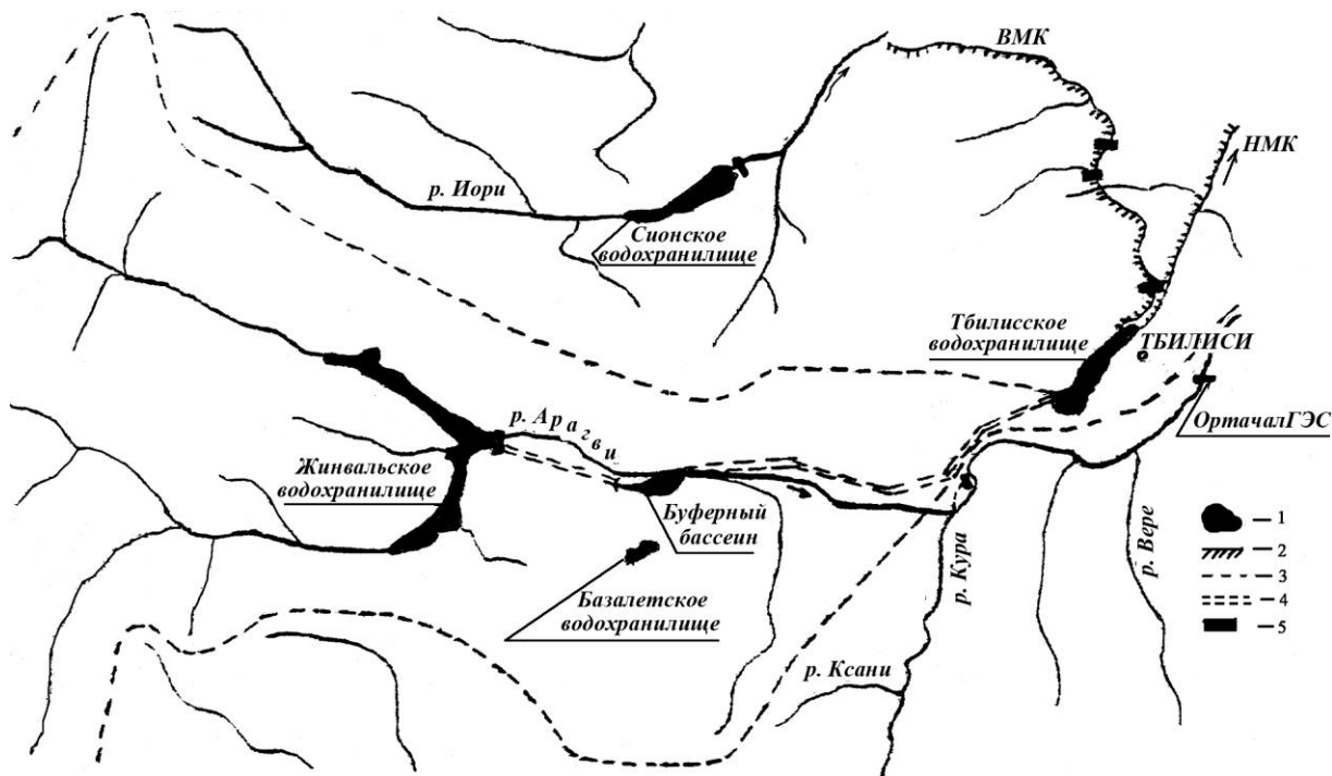
Рис. 4.2.5. Схема совместной работы Сионского, Тбилисского и Жинвальского водохранилищ: 1 – водохранилища; 2 – каналы; 3 – водораздел бассейнов рек; 4 – водоводы; 5 – ГЭС
