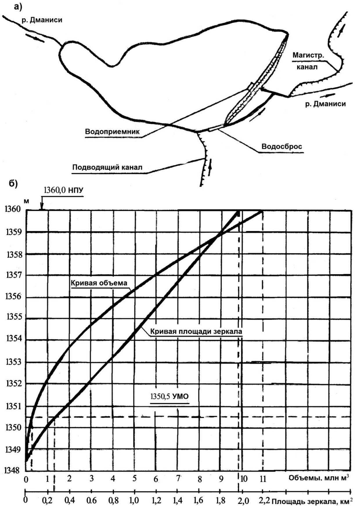
Рис. 4.2.18. Дманисское (Якублойское) водохранилище: а) схема водохранилищной системы; б) график площади зеркала и объема водохранилища
