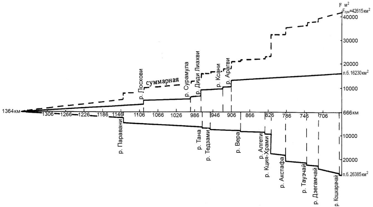
Рис. 4.1.2. График увеличения площади бассейна р. Кура от истока до Мингечевирского водохранилища
