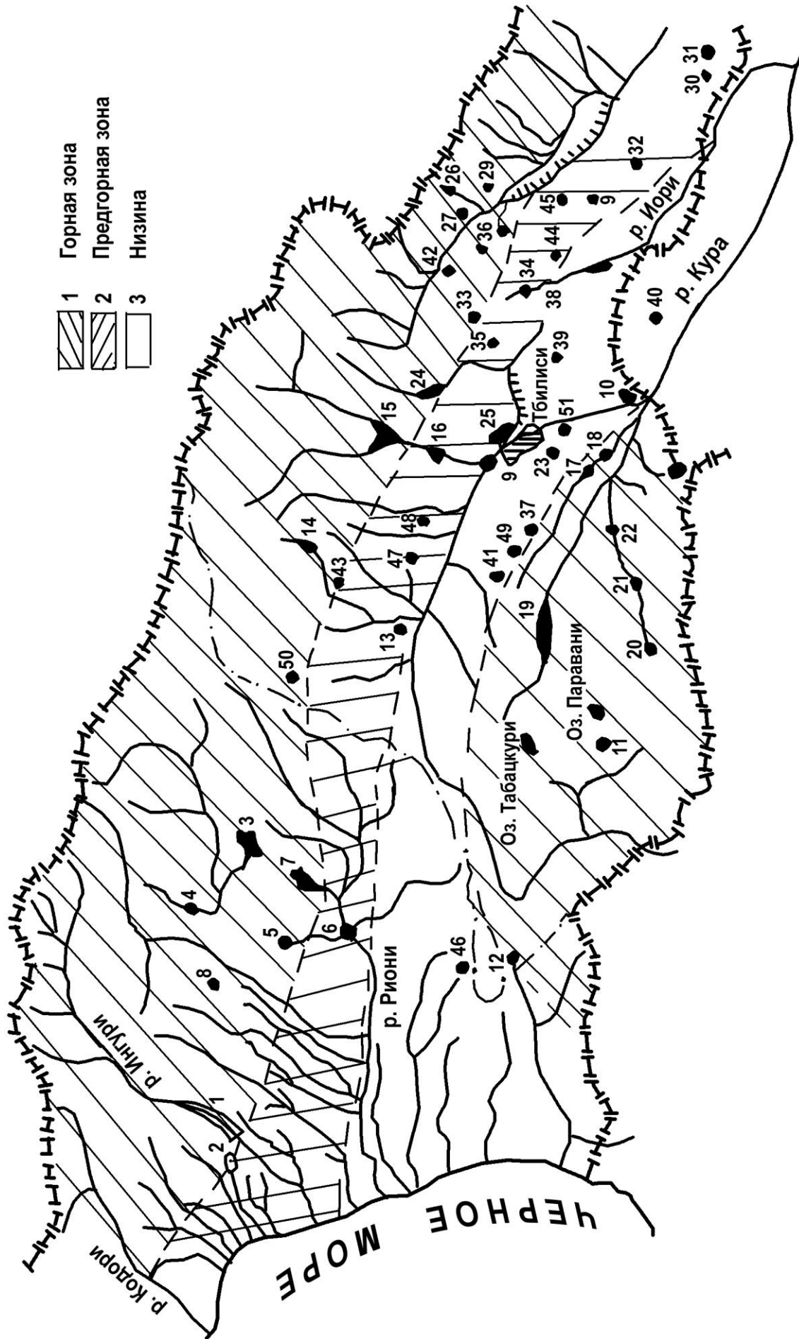
Рис. 4.2.1-б. Расположение всех водохранилищ Грузии (Название водохранилищ с соответствующей нумерацией приведено в табл. 4.2.1)
