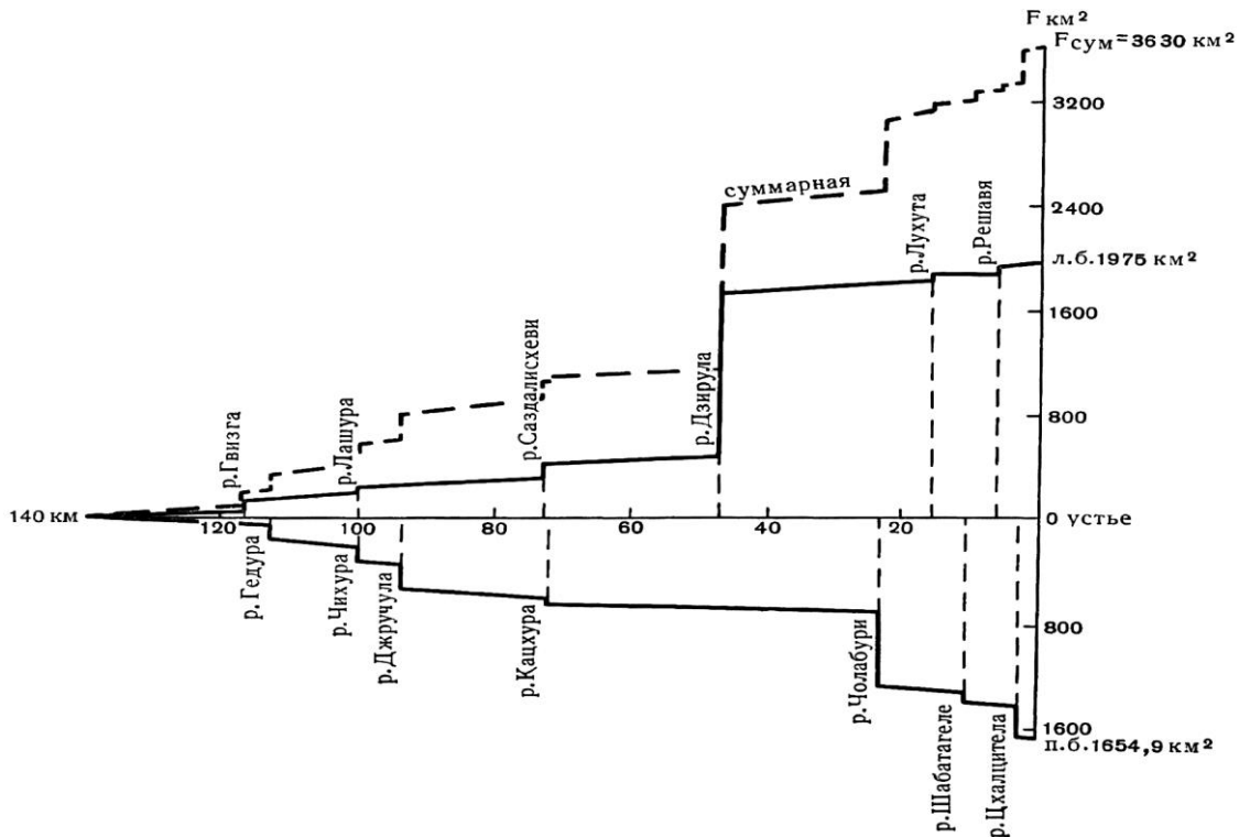
Рис. 4.1.36. График увеличения площади бассейна р. Квирила
