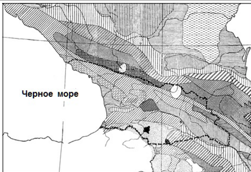
Рис. 3.2. Карта геоморфологического районирования Грузии
