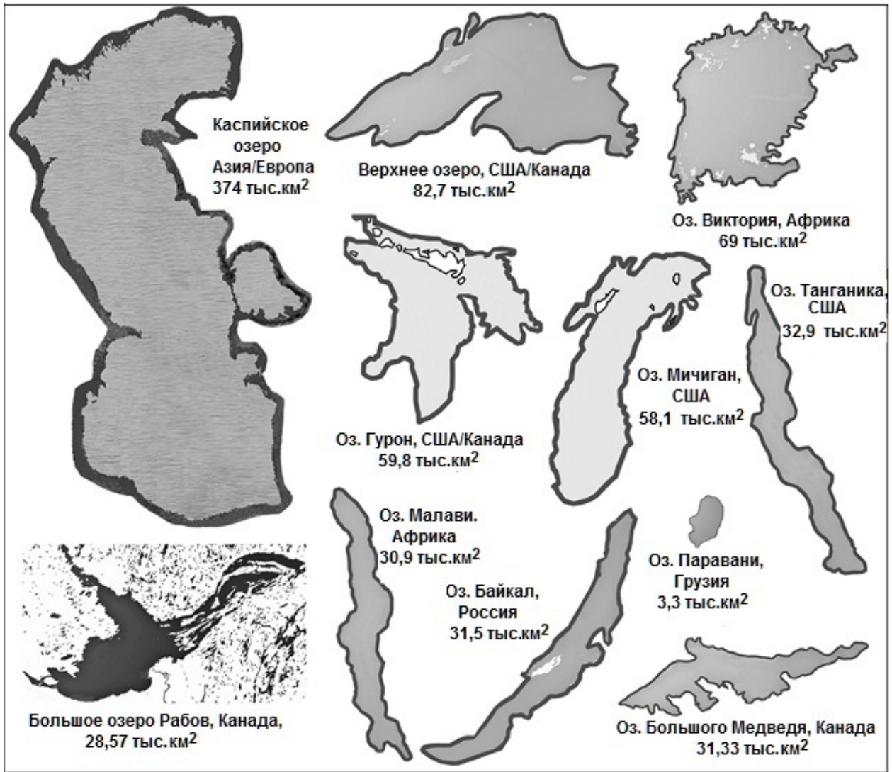
Рис. 1.4.1. Крупнейшие озера Мира
