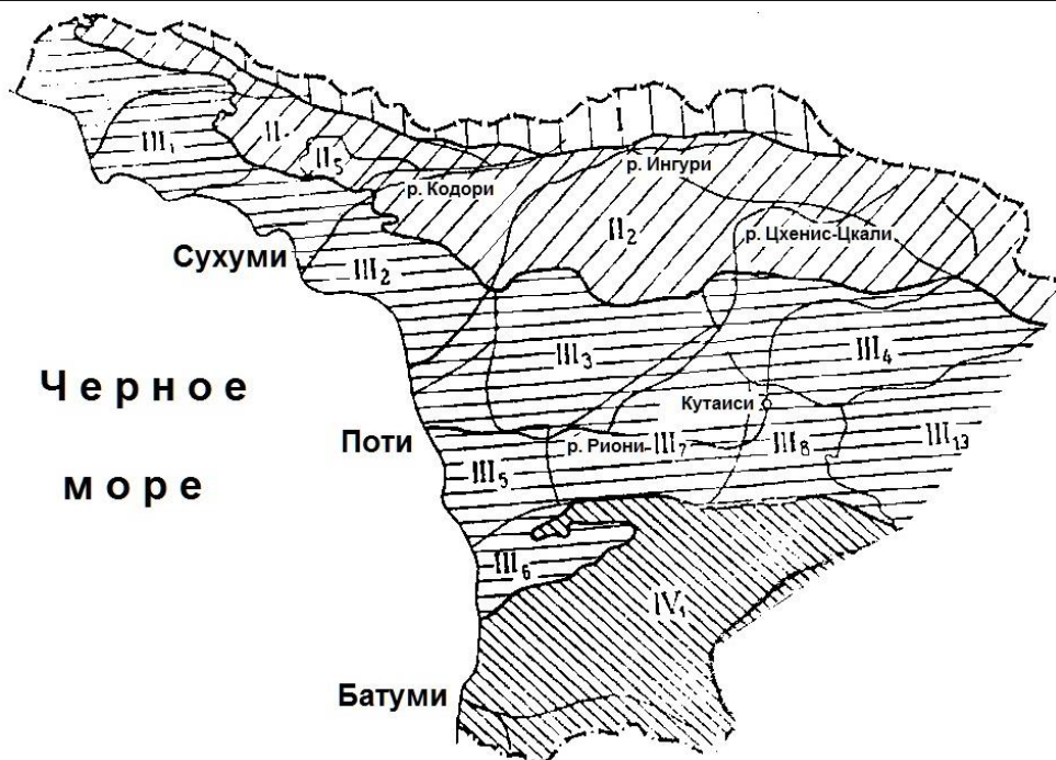
Рис. 4.2.61. Районирование подземных вод Западной Грузии:
