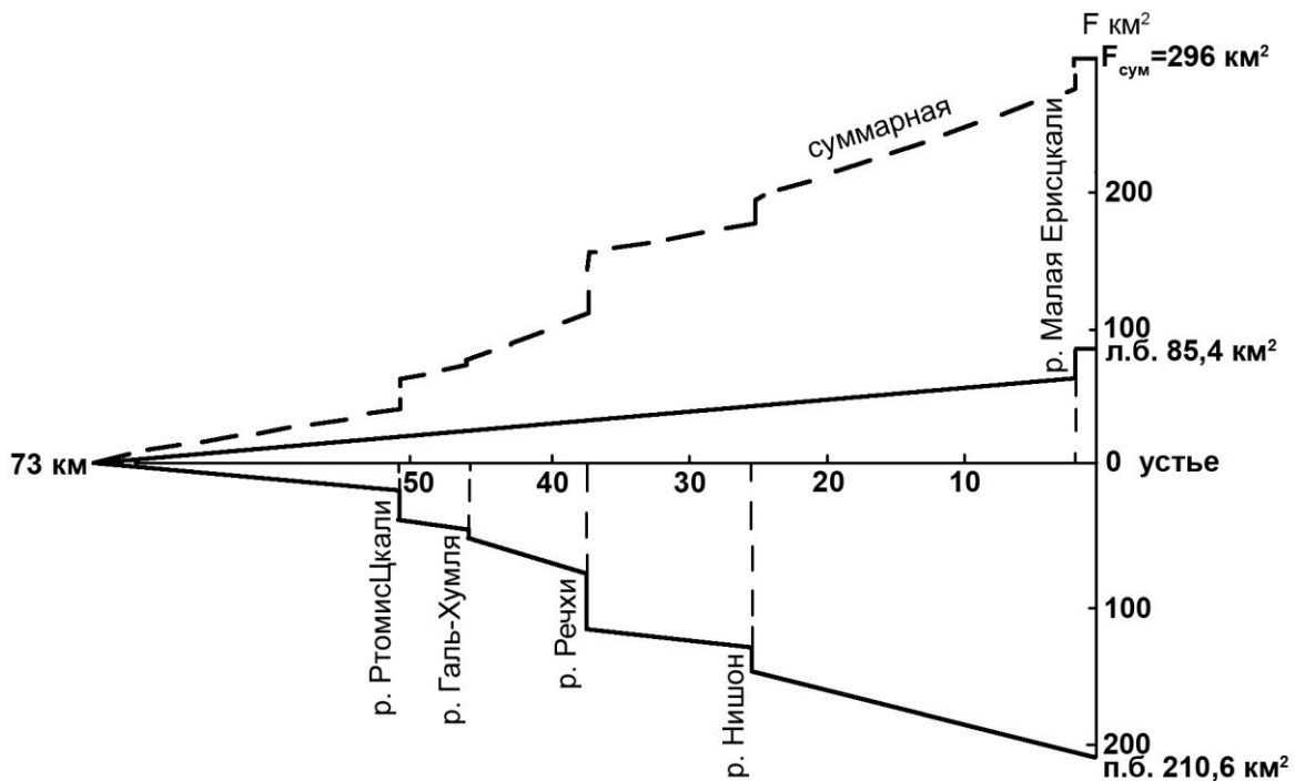
Рис. 4.1.26. График увеличения площади бассейна р. Диди Эрис-Цкали
