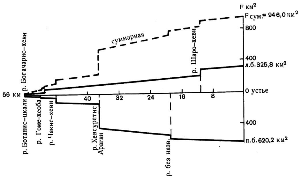
Рис. 4.1.9. График увеличения площади бассейна р. Араги
