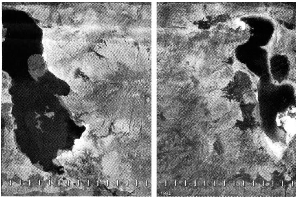
Рис. 1.4.2. Динамика высыхания озера Урмия (космическая аэрофотосъемка)
