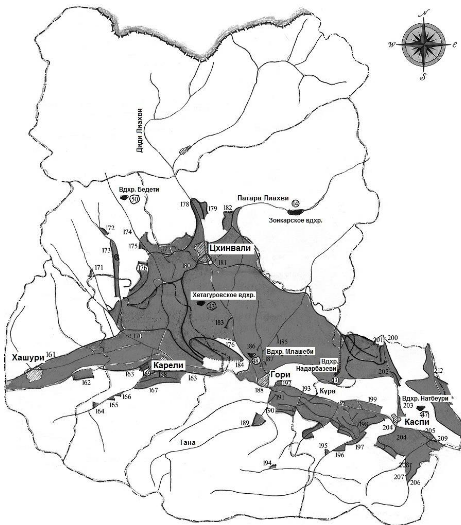
Рис. 4.2.2-к. Гидромелиоративная карта Шиди Картли
