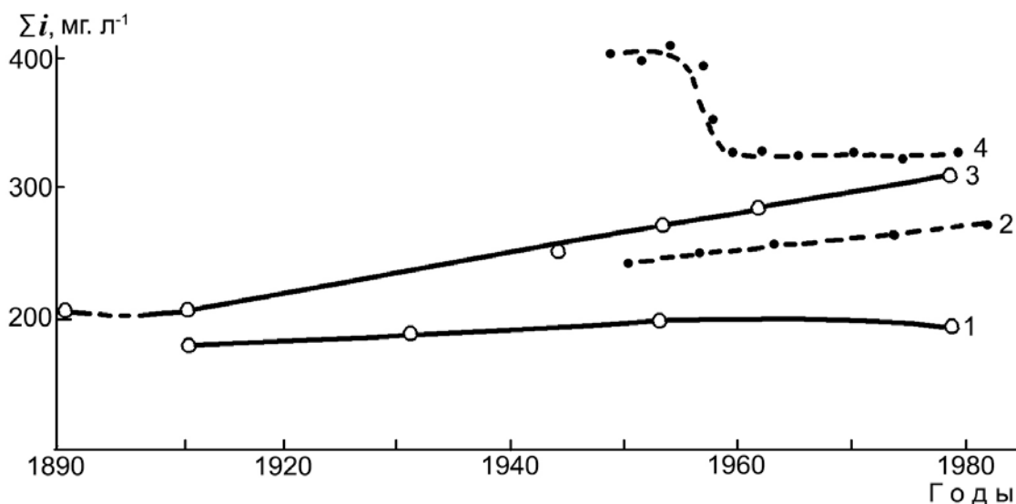
Рис. 7.3. Изменение суммы главных ионов \sum i воды во времени: 1 - р. Риони, 2 - р. Арагви, 3 - р. Кура, 4 - Тбилисское водохранилище.
