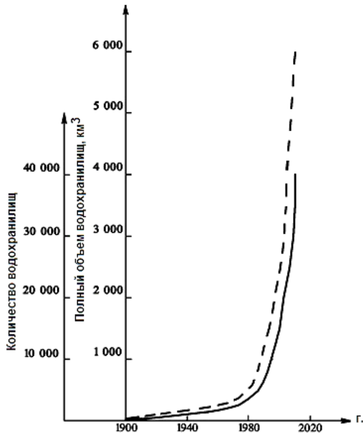
Рис. 1.3.1. Динамика роста количества и полного объема водохранилищ объемом более 1 млн. м 3 в мире
