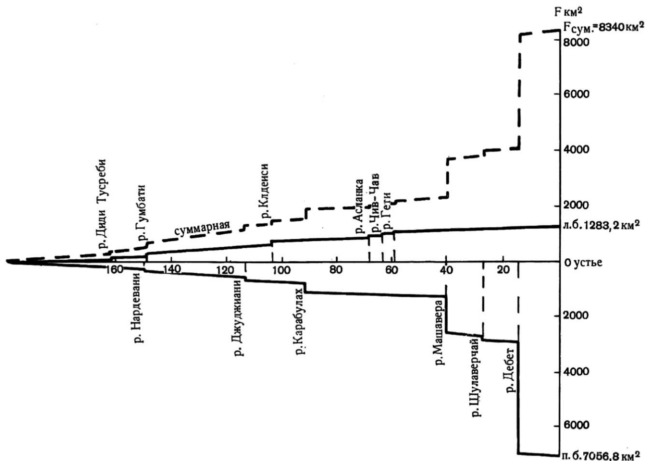
Рис. 4.1.6. График увеличения площади бассейна р. Храми
