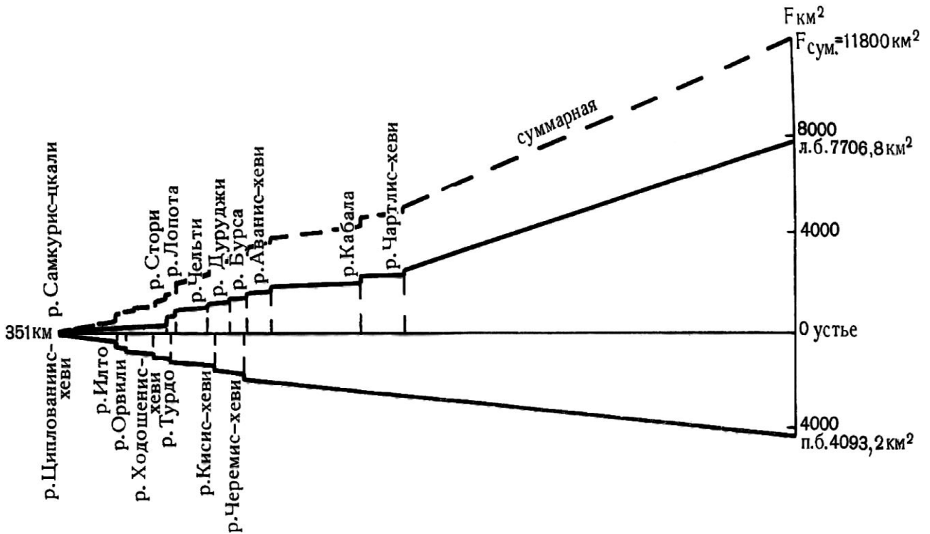
Рис. 4.1.4. График увеличения площади бассейна р. Алазани
