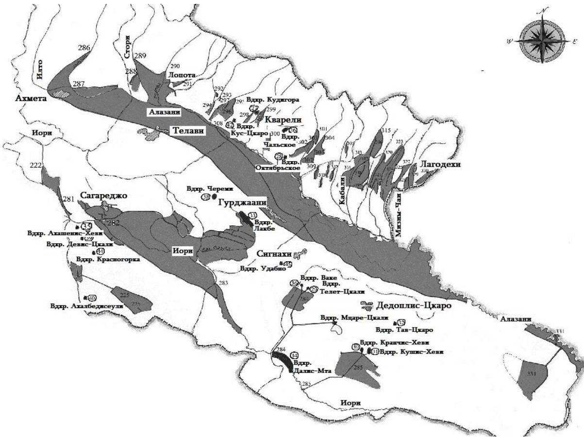
Рис. 4.2.2 - ж. Гидромелиоративная карта Кахети
