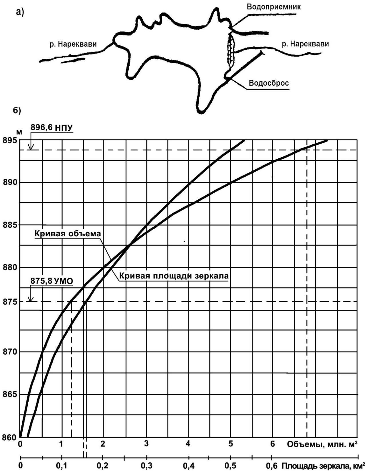
Рис. 4.2.24. Нареквавское водохранилище а) схема водохранилищной системы; б) график площади зеркала и объема водохранилища
