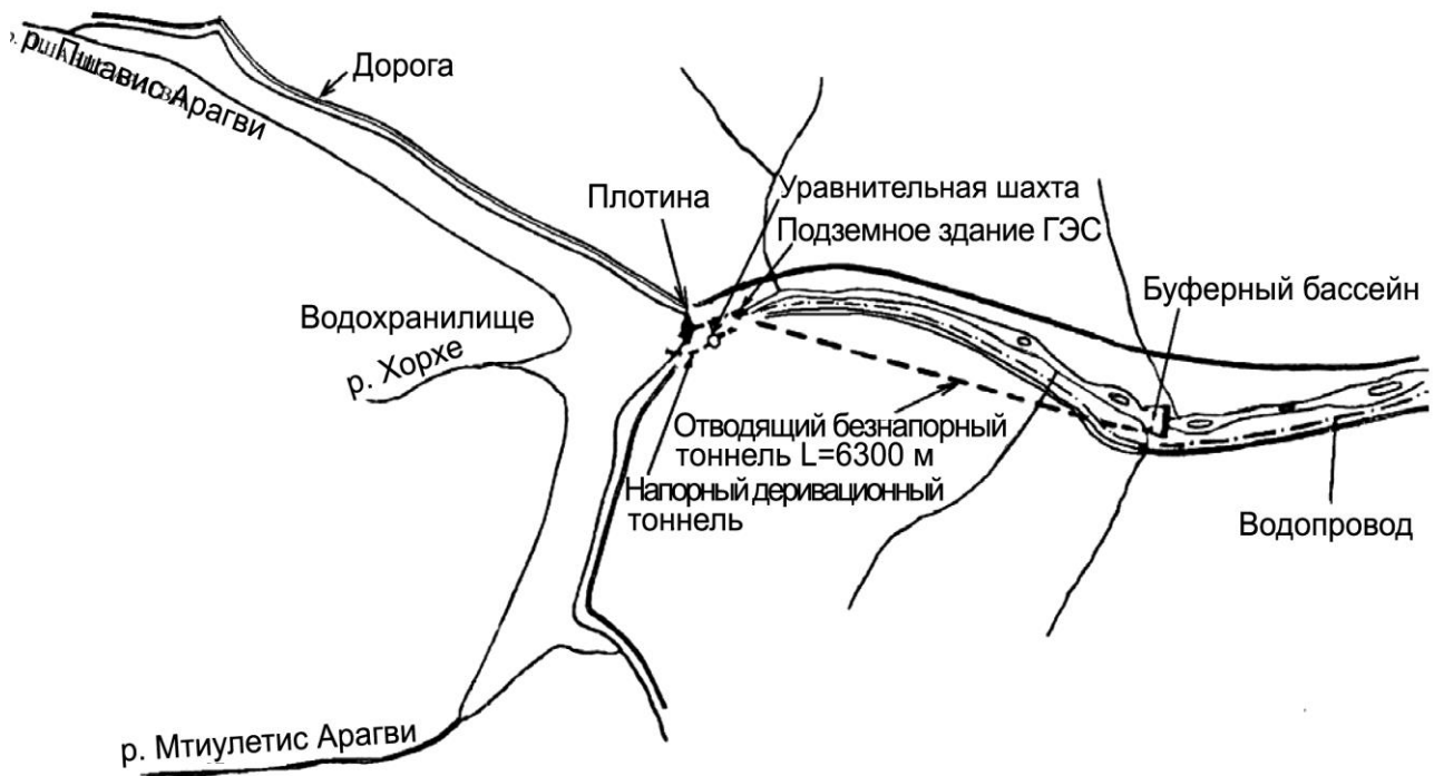
Рис. 4.2.27. Схема Жинвальской водохранилищной системы
