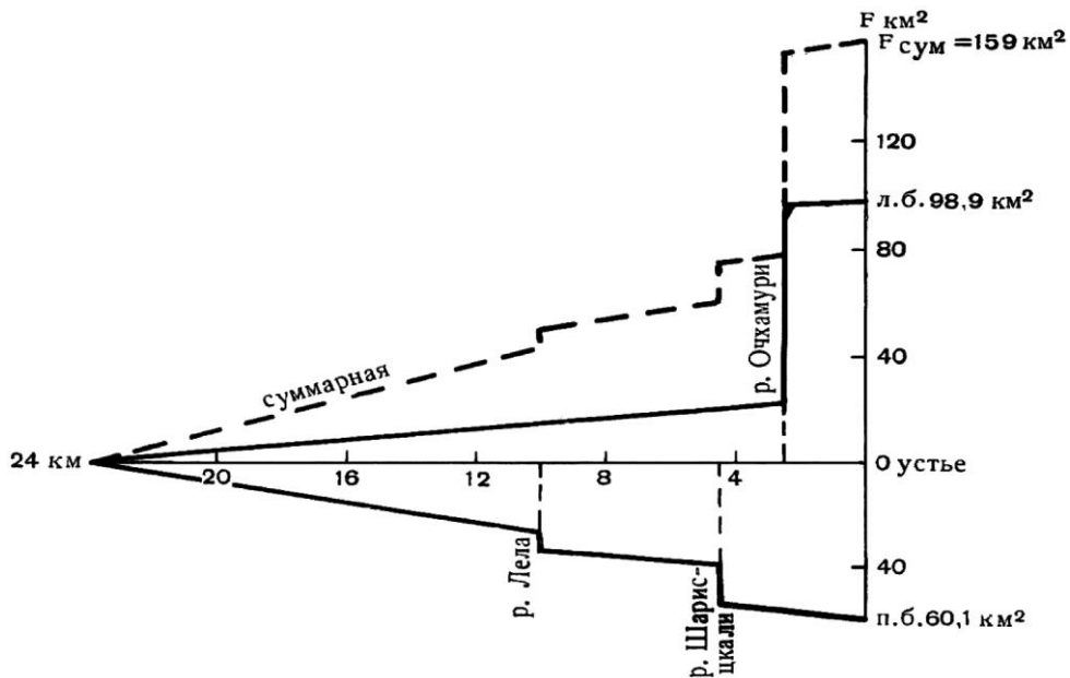
Рис. 4.1.48. График роста площади бассейна р. Чолоки
