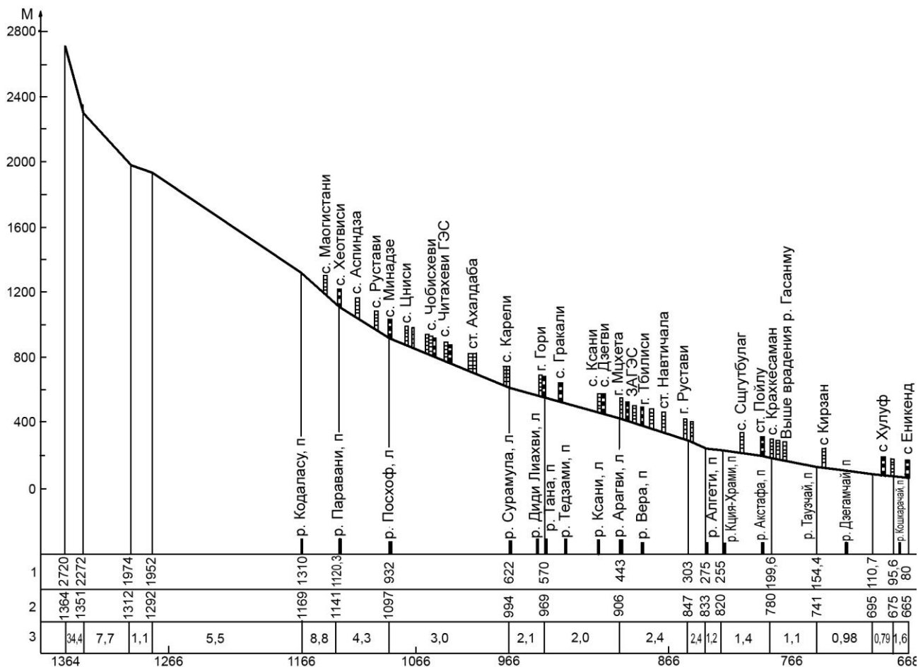
Рис. 4.1.1. Продольный профиль р. Куры от истока до Мингечевириского водохранилища
