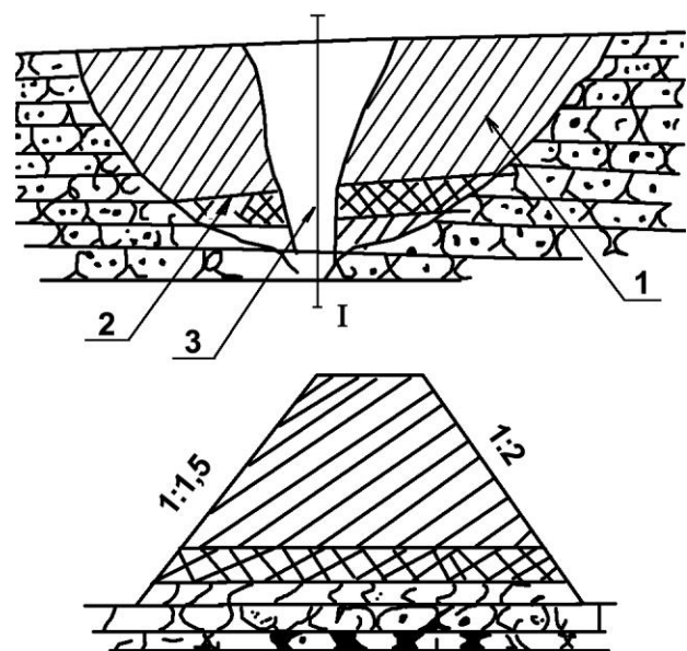
Рис. 4.2.52. Разрушение плотины в Даба Цкнети (1980 г.)
