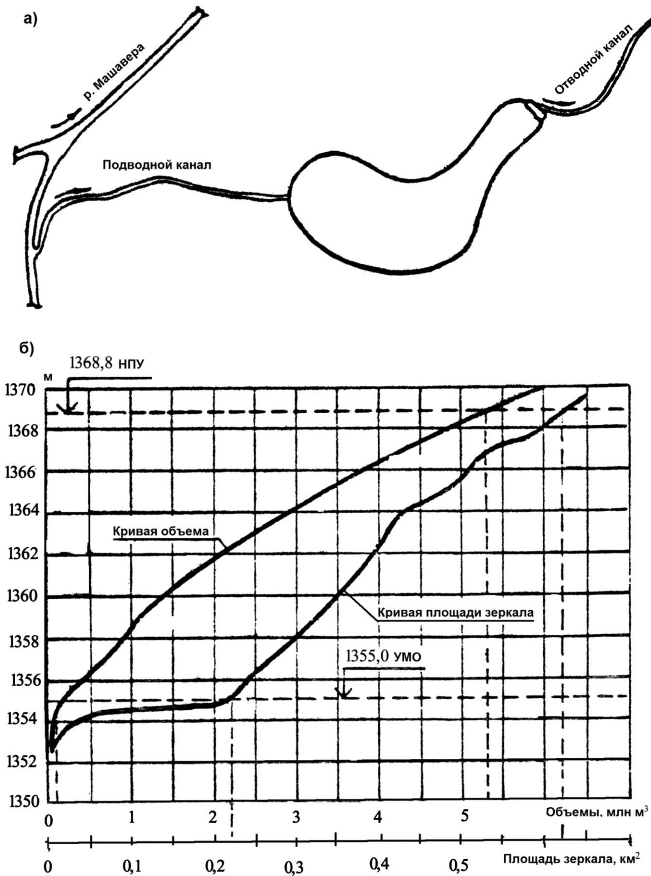
Рис. 4.2.25. Пантианское водохранилище: а) схема водохранилищной системы; б) график площади зеркала и объема водохранилища
