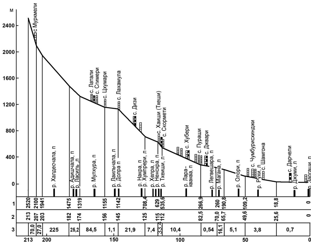
Рис. 4.1.27. Схематический продольный профиль р. Ингури
