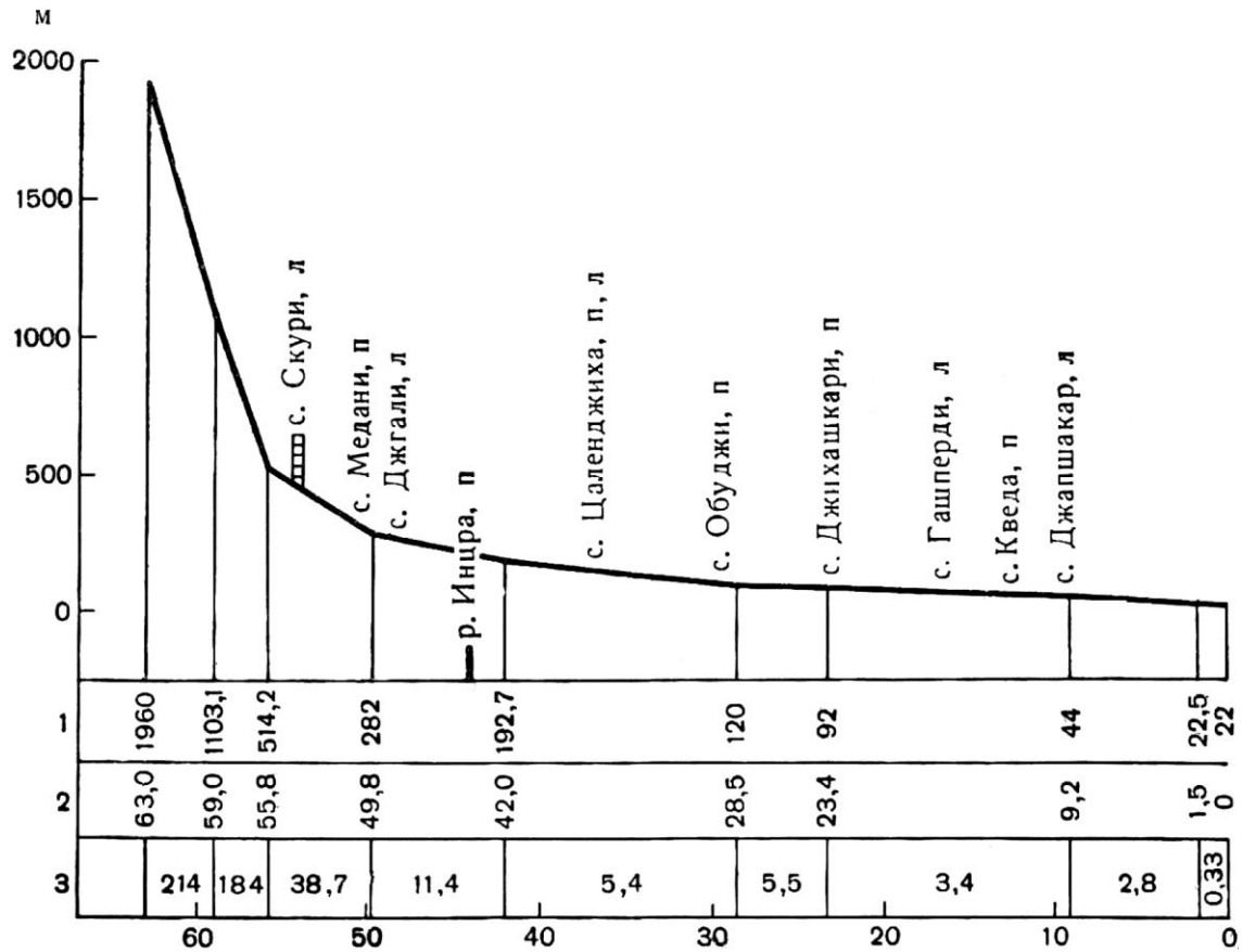
Рис. 4.1.31. Схематический продольный профиль р. Чанис-Цкали
