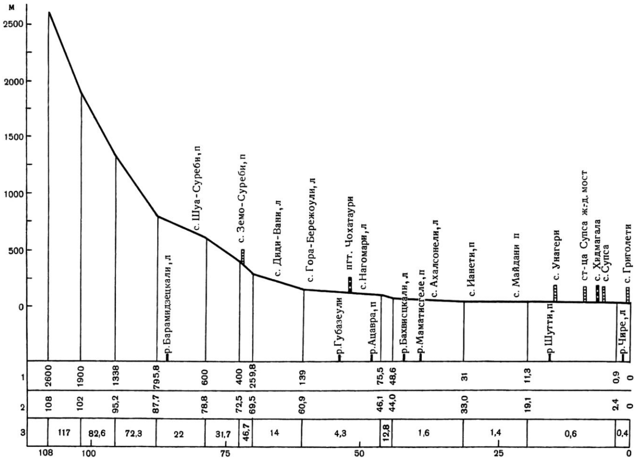
Рис. 4.1.43. Схематический продольный профиль р. Супса
