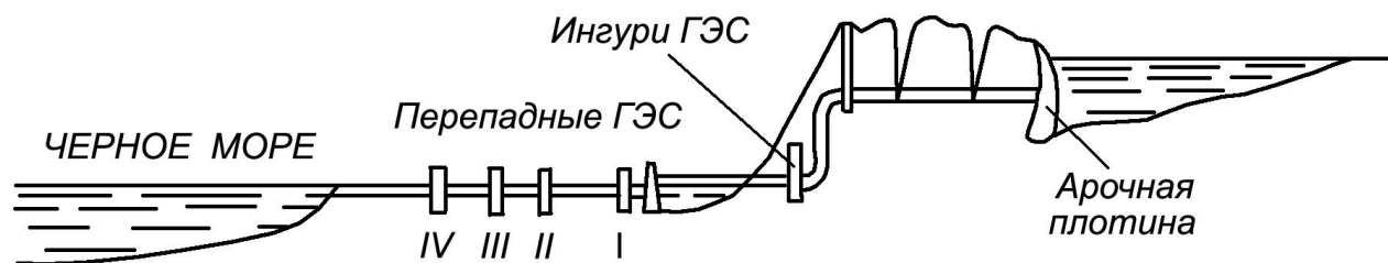
Рис. 4.2.30. Общая схема расположения гидротехнических сооружений на Ингури ГЭС 1 – отводящий канал; 2 – перепадная ГЭС IV; 3 – перепадная ГЭС III; 4 – перепадная ГЭС II; 5 – перепадная ГЭС I; 6 – плотина перепадной ГЭС I; 7 – отводящий канал; 8 – открытое распределительное устройство – 500 кВт; 9 – подземное здание Ингури ГЭС; 10 – уравнильный резервуар; 11 – деривационный тоннель; 12 – арочная плотина; 13 – сбросные сооружения стока р. Ингури в р. Эрис-Цкали (водосливная плотина, водоприемный шлюз); 14 – каналы №1 и №2; 15 – безнапорный туннель
