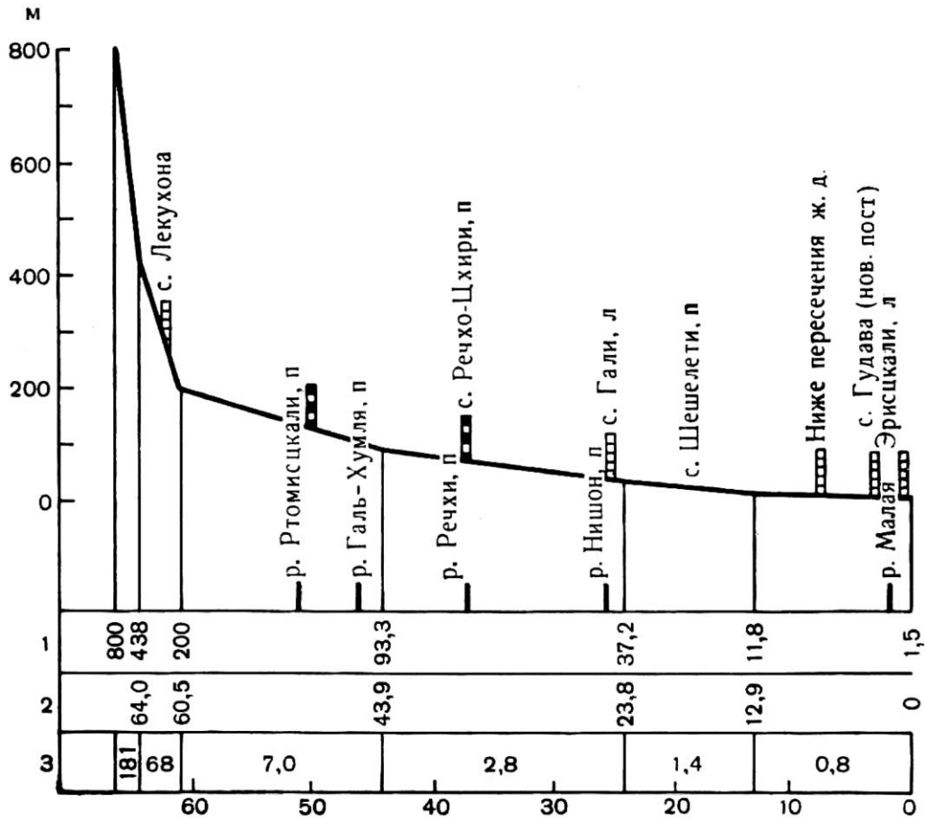
Рис. 4.1.23. Схематический продольный профиль р. Галидзга
