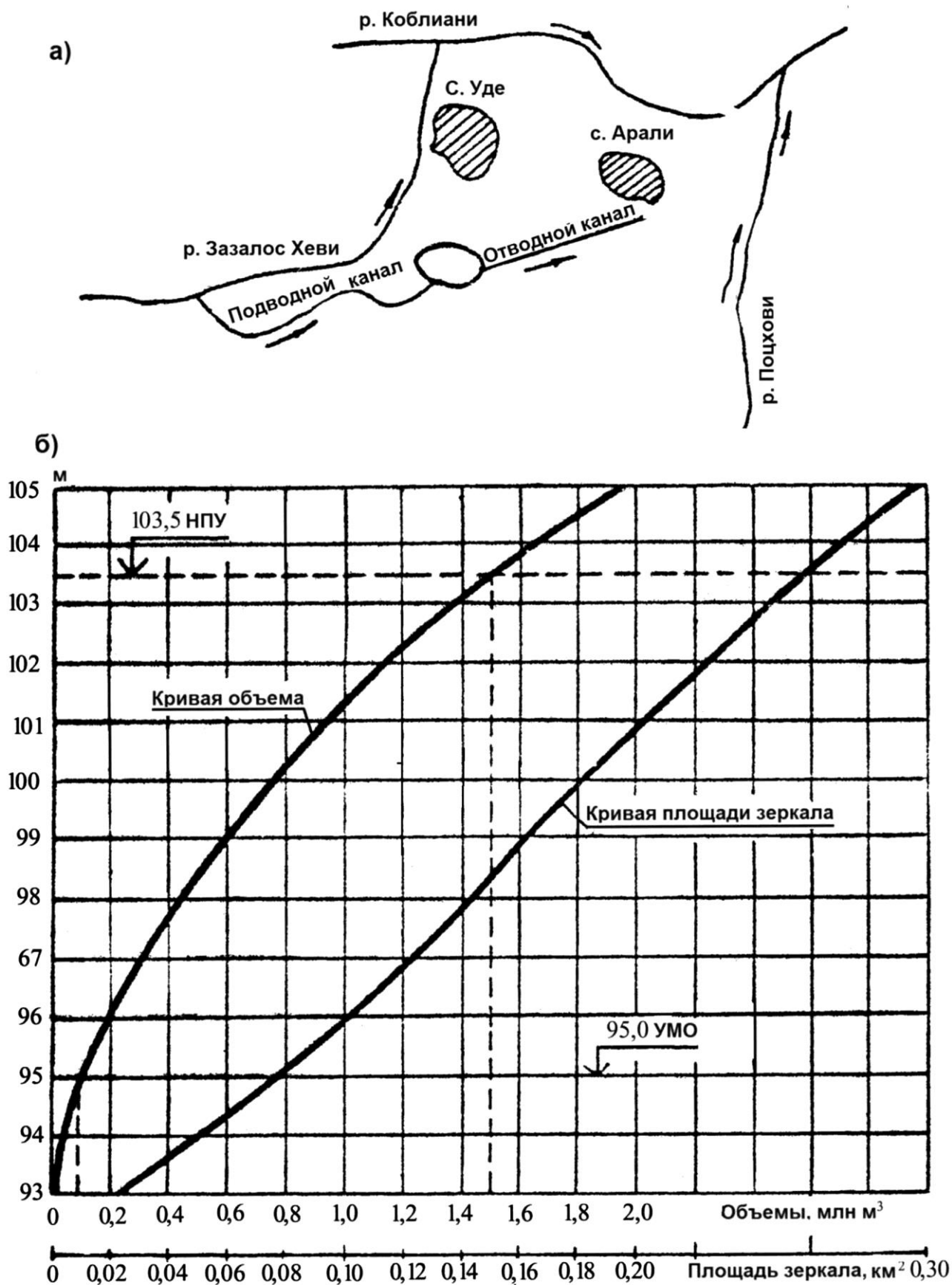
Рис. 4.2.15. Цхенисис-Чисское (Уде) водохранилище: а) схема водохранилищной системы; б) график площади зеркала поверхности и объема водохранилища
