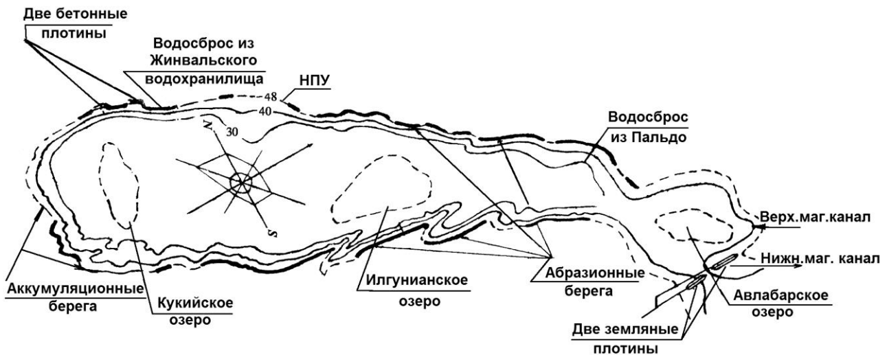
Рис. 4.2.51. Гидротехнические сооружения Тбилисского водохранилища
