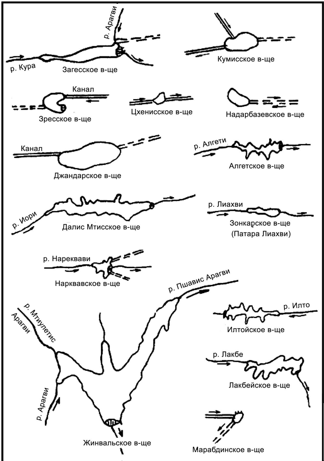
Рис. 4.2.3-б. Формы водохранилищ Восточной Грузии (в соотносительном масштабе)
