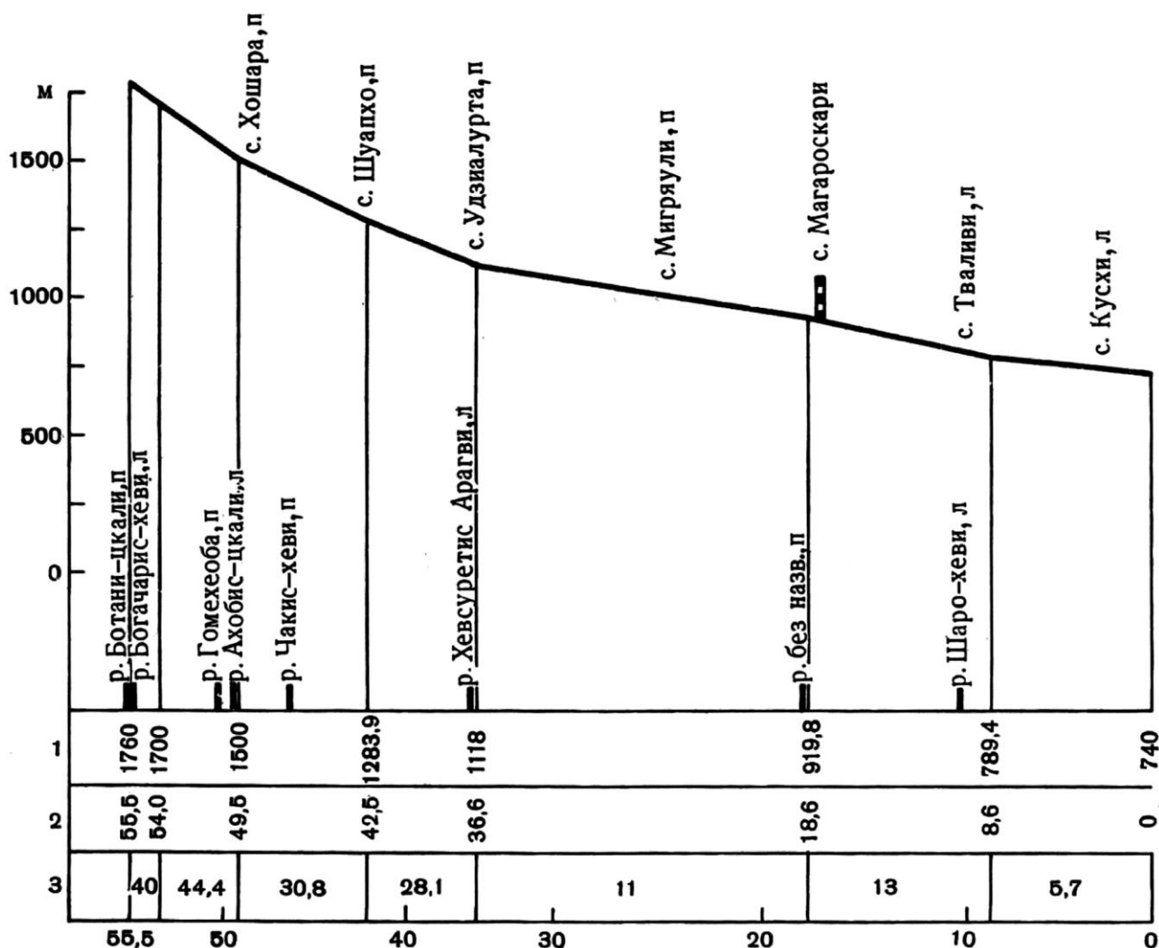
Рис. 4.1.10. Продольный профиль р. Арагви
