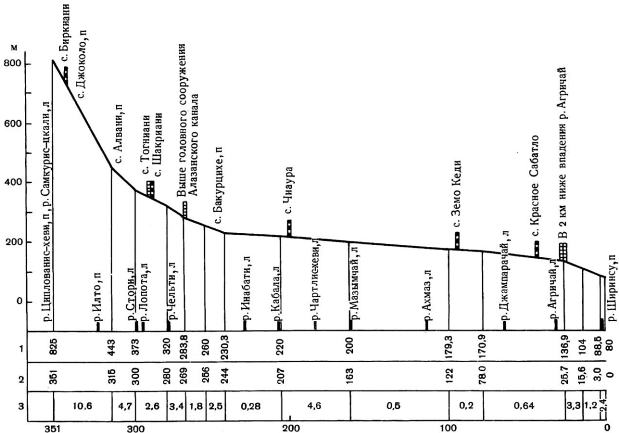
Рис. 4.1.3. Продольный профиль р. Алазани
