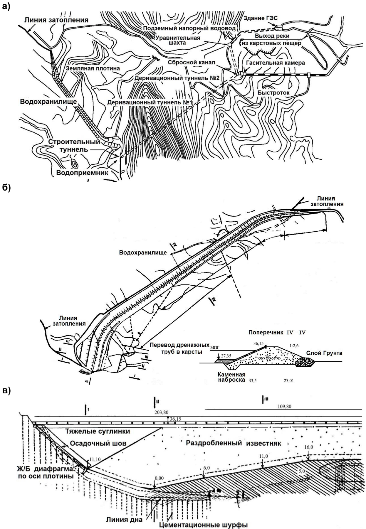
Рис. 4.2.50. Головной узел Ткибульского водохранилища: а) план гидроузла; б) план плотины; в) продольный профиль плотины
