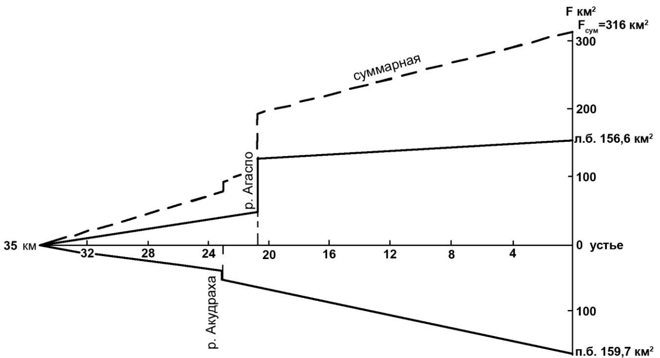
Рис. 4.1.16. График увеличения площади водосбора р. Западной Гумисты
