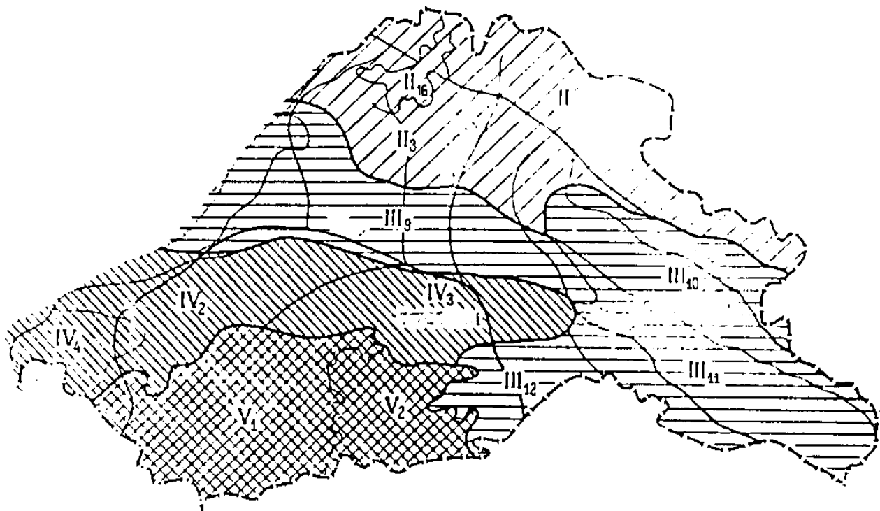
Рис. 4.2.59. Районирование подземных вод Восточной Грузии.
