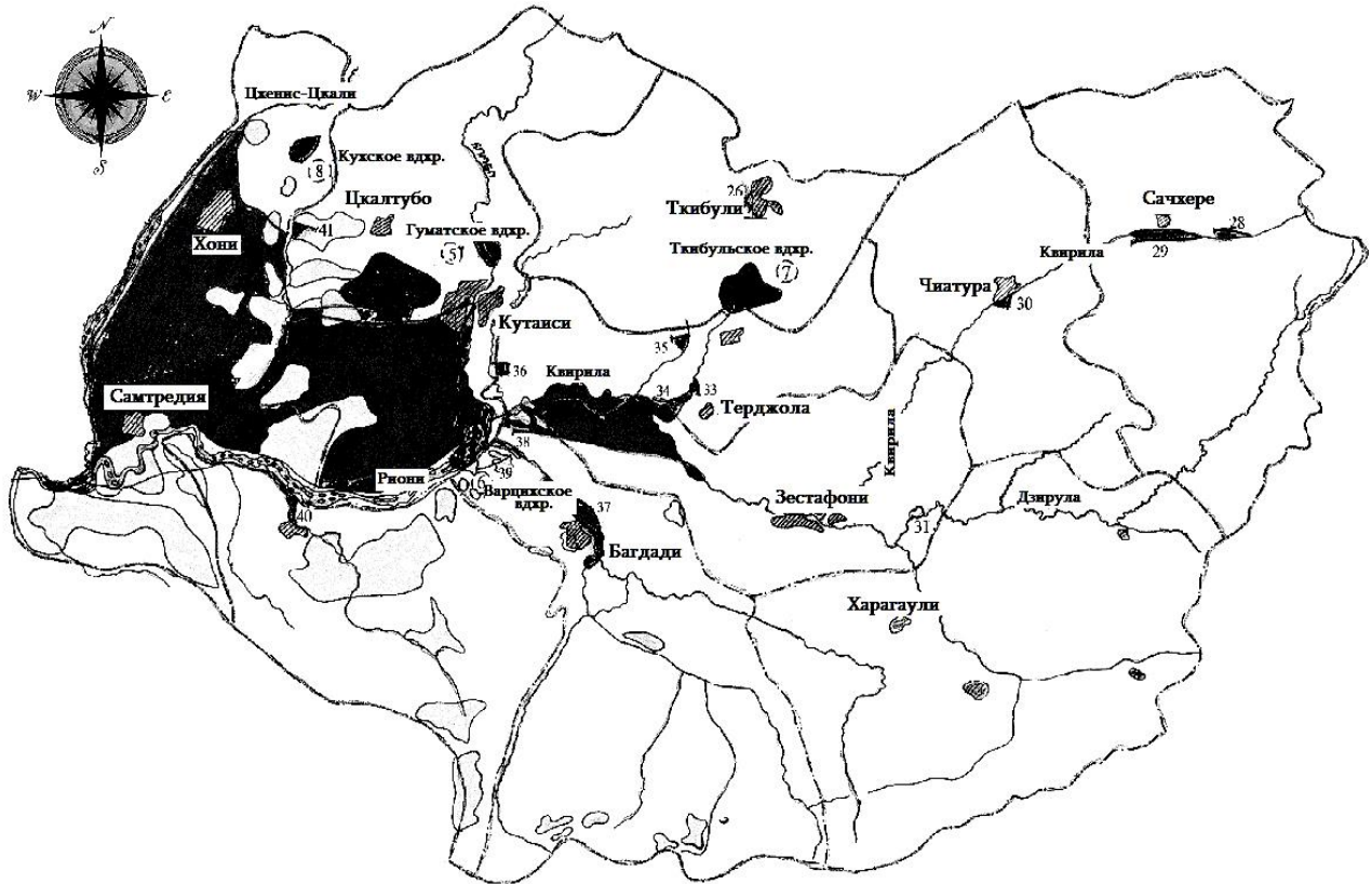
Рис. 4.2.2-д. Гидромелиоративная карта Имерети
