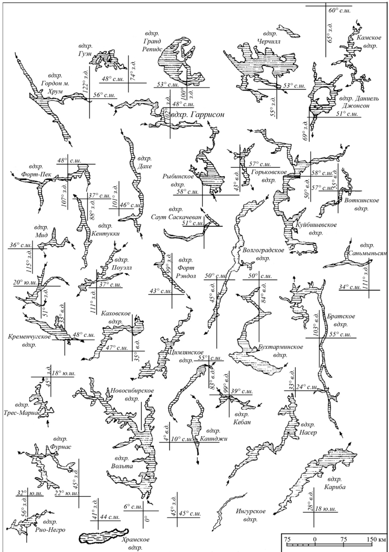
Рис. 1.3.3. Конфигурация зеркала поверхности ряда крупных водохранилищ мира (Цифрами обозначена географическая широта и долгота)
