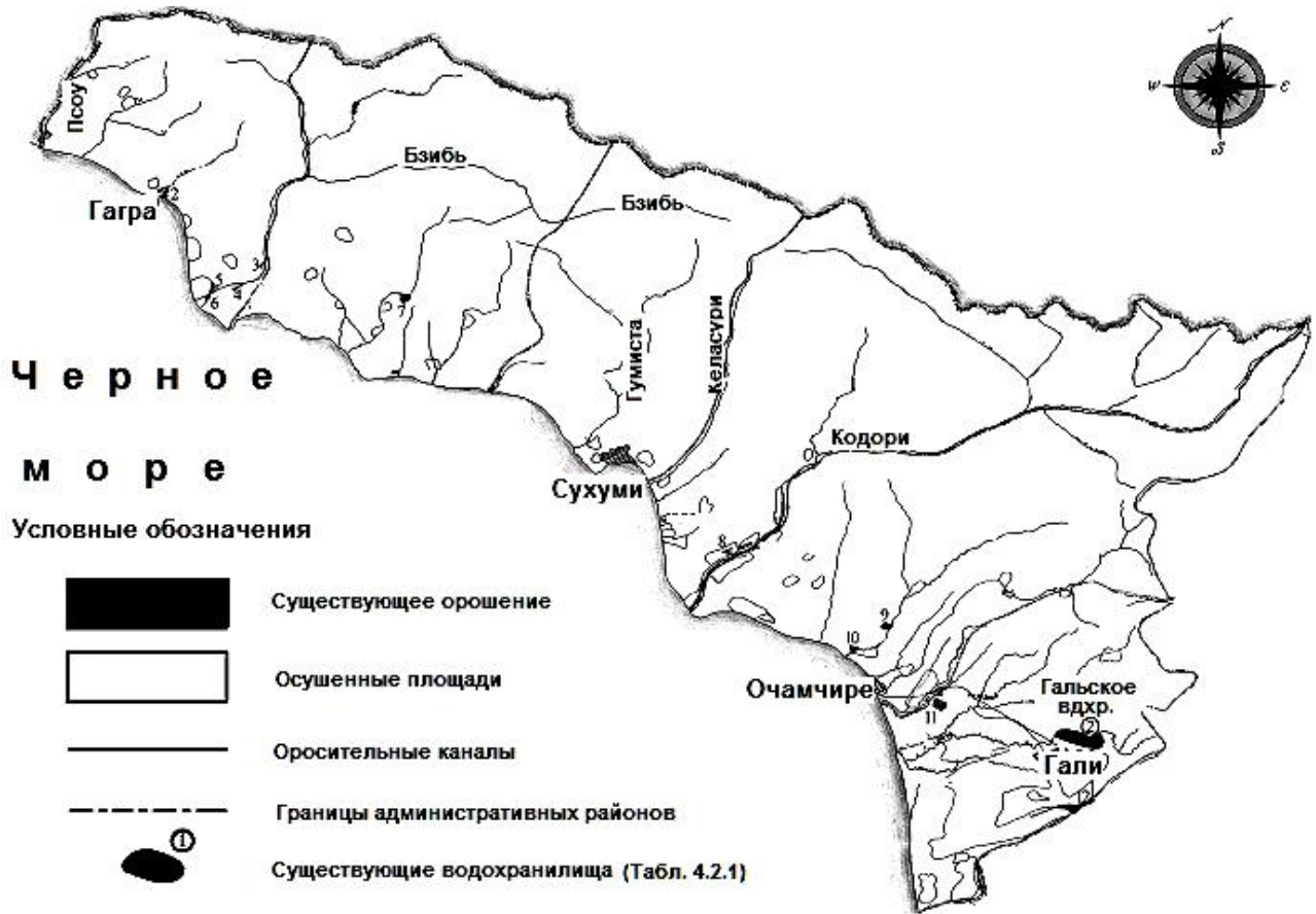
Рис. 4.2.2-а. Гидромелиоративная карта Абхазии
