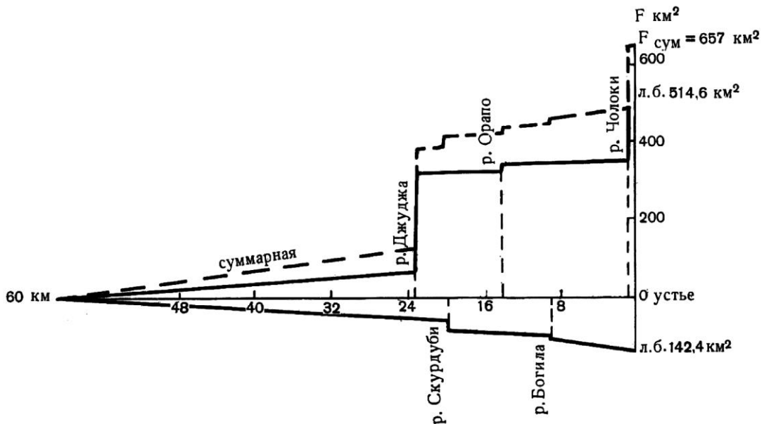
Рис. 4.1.46. График роста площади бассейна р. Натанеби
