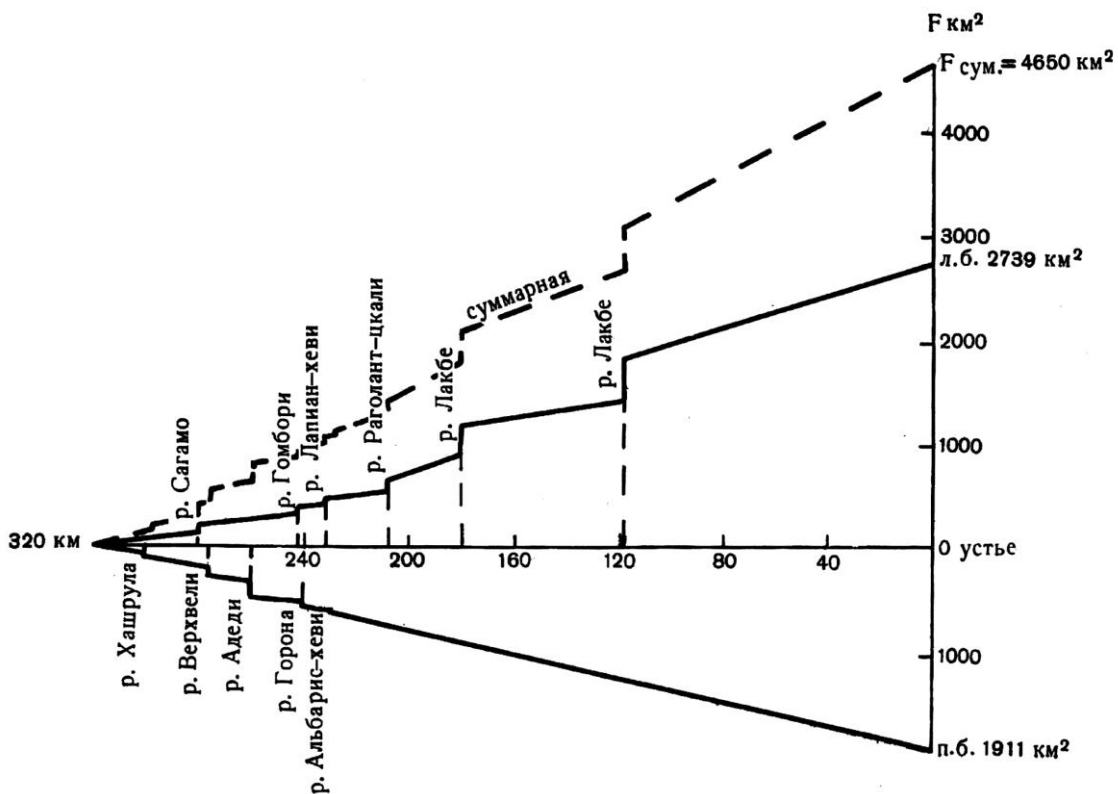
Рис. 4.1.7. График увеличения площади бассейна р. Иори
