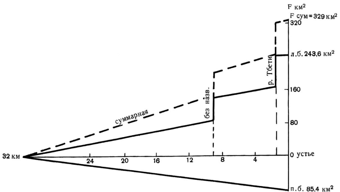
Рис. 4.1.50. График роста площади бассейна р. Чирухис-Цкали
