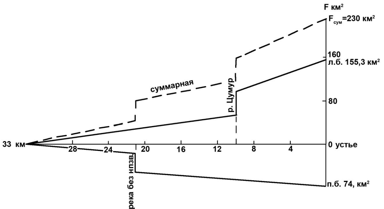
Рис. 4.1.18. График увеличения площади бассейна р. Восточной Гумисты
