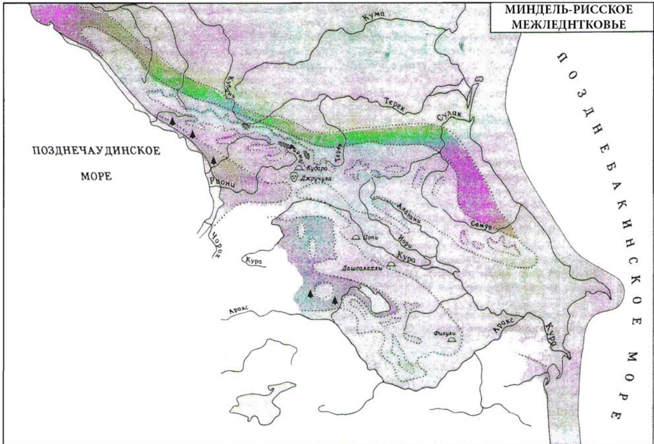
Рис. 2.1. Развитие бассейнов Чёрного и Каспийского морей (Верхний Олигоцен – Миндель-Рисское межледниковье)
