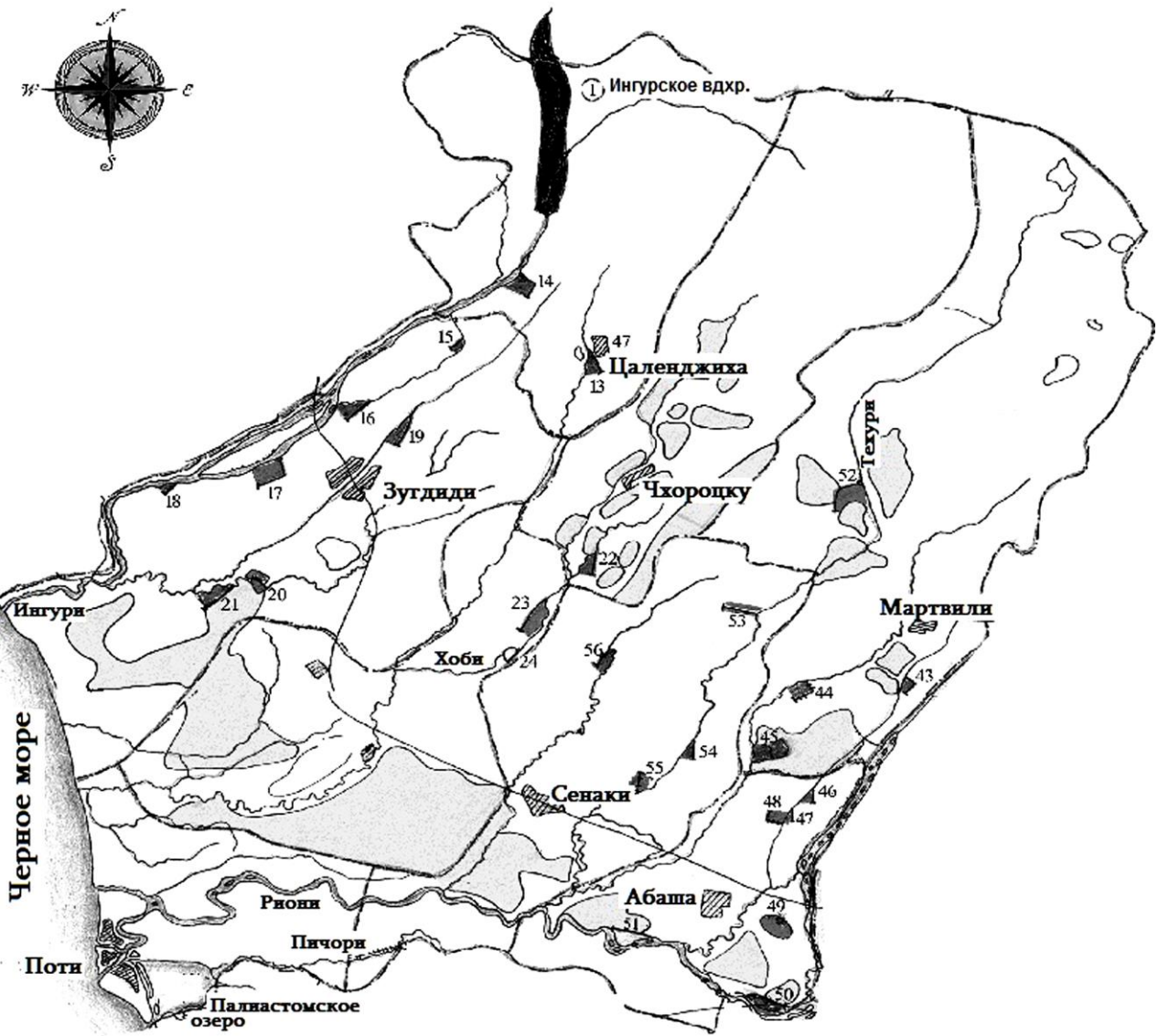
Рис. 4.2.2-г. Гидромелиоративная карта Самегрело
