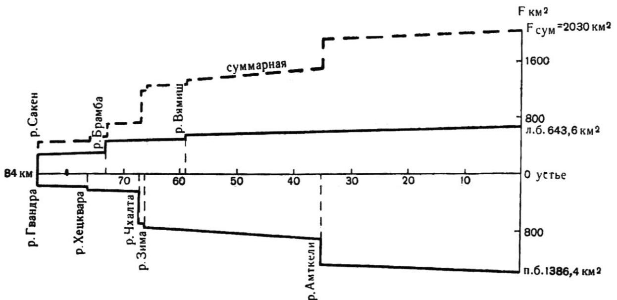
Рис. 4.1.20. График увеличения площади бассейна р. Кодори
