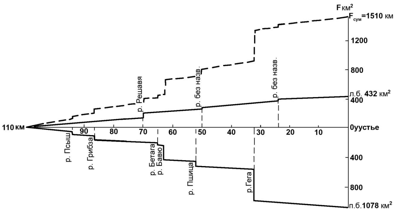
Рис. 4.1.14. График увеличения площади бассейна р. Бзыбь
