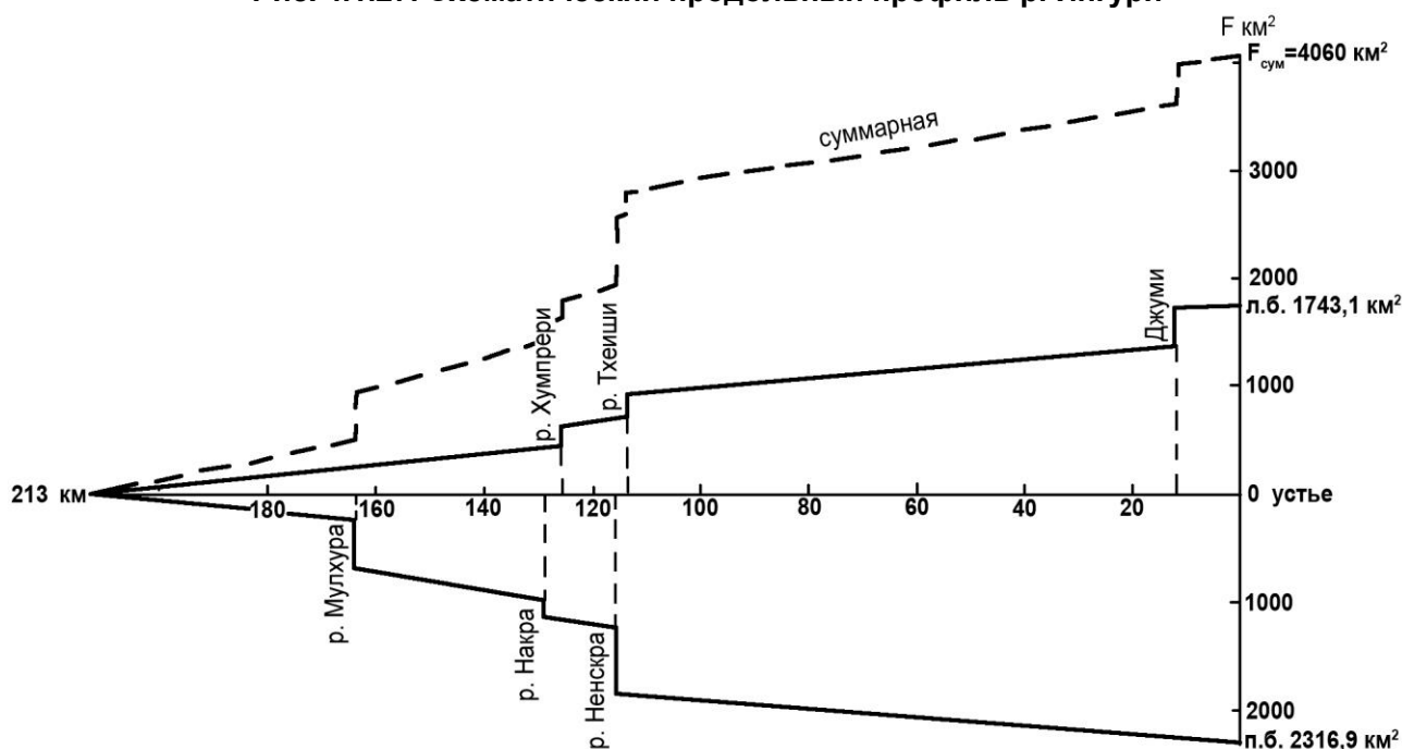
Рис. 4.1.28. График увеличения площади бассейна р. Ингури
