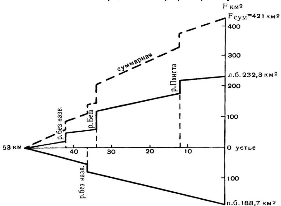
Рис. 4.1.12. График увеличения площади бассейна р. Псоу
