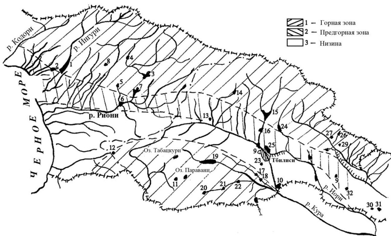
Рис. 4.2.1-а. Расположение водохранилищ Грузии (объемом >1млн м 3 ) (Название водохранилищ с соответствующей нумерацией приведено в табл. 4.2.1)
