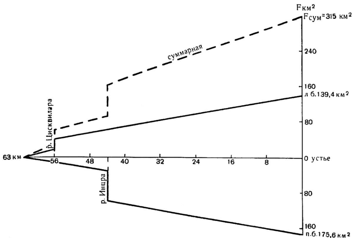
Рис. 4.1.32. График увеличения площади бассейна р. Чанис-Цкали
