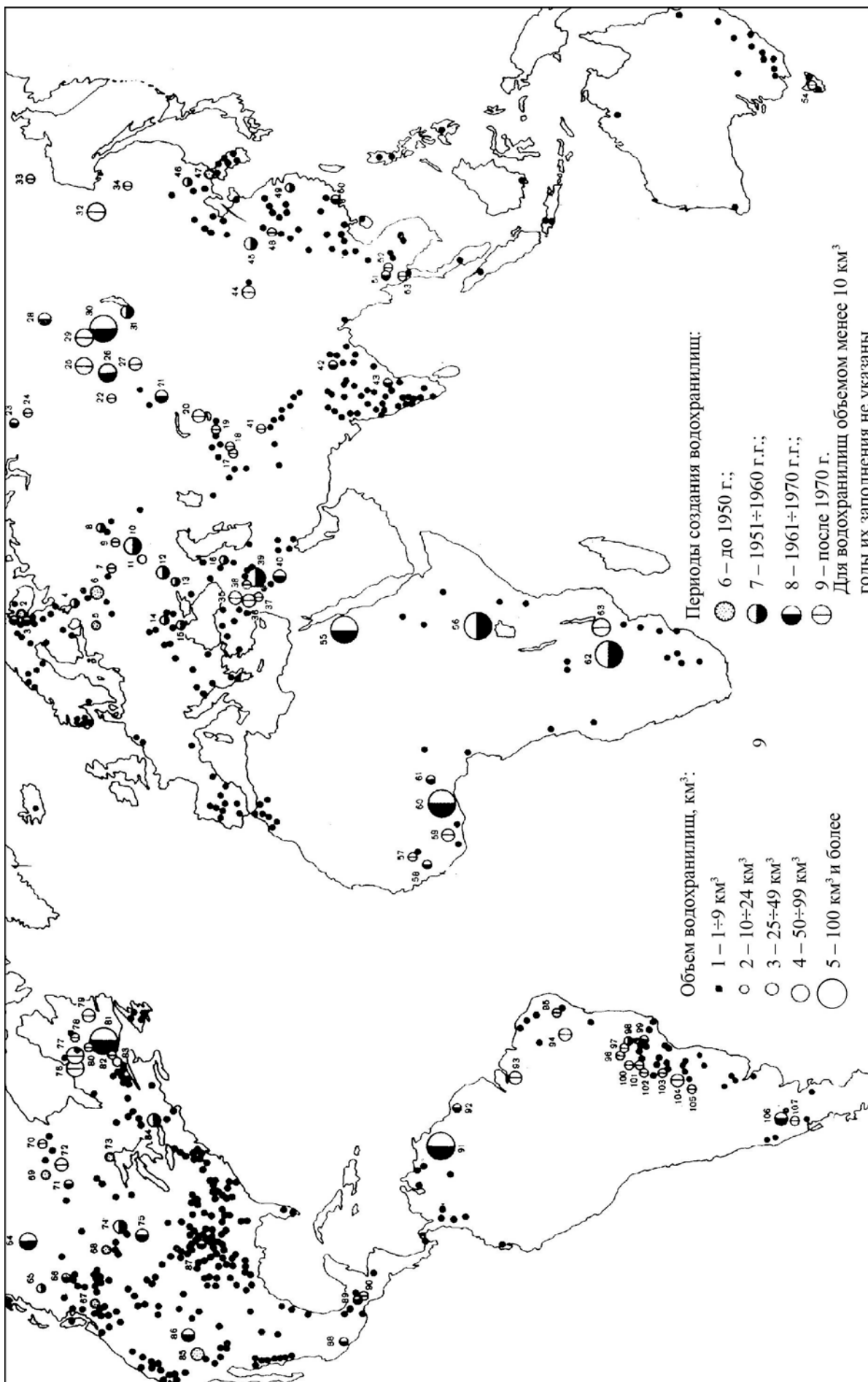
Рис. 1.3.2. Схема расположения водохранилищ мира объемом более 1 км 3
