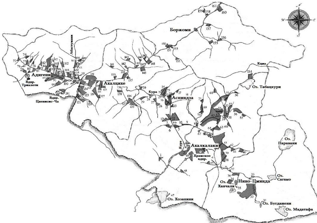
Рис. 4.2.2-з. Гидромелиоративная карта Самцхе-Джаваheti
