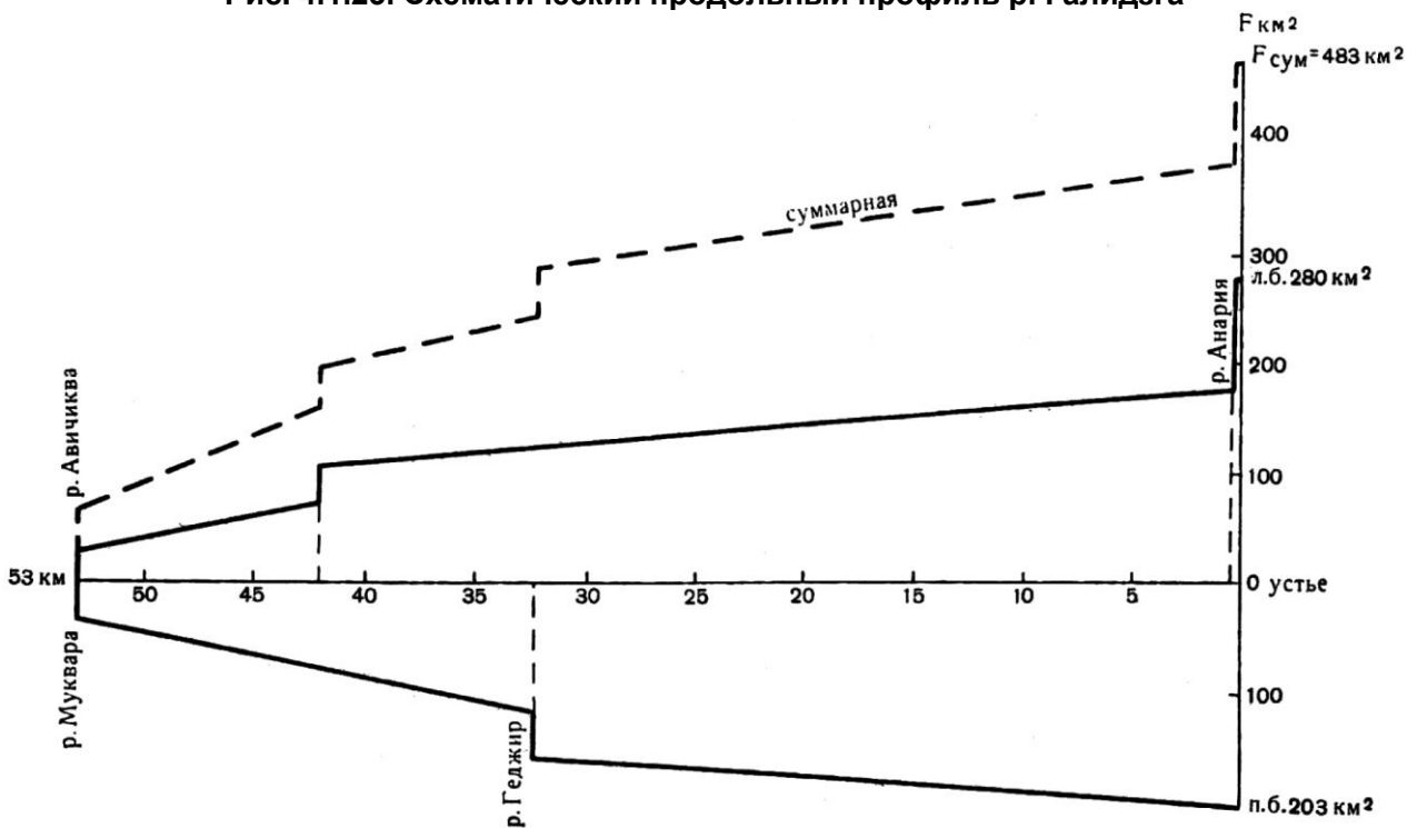
Рис. 4.1.24. График увеличения площади бассейна р. Галидзга
