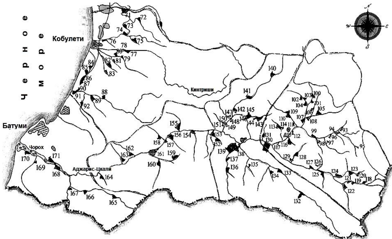
Рис. 4.2.2-б. Гидромелиоративная карта Аджарии
