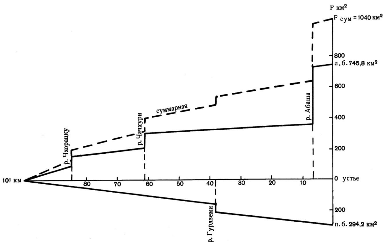
Рис. 4.1.42. График роста площади бассейна р. Техура
