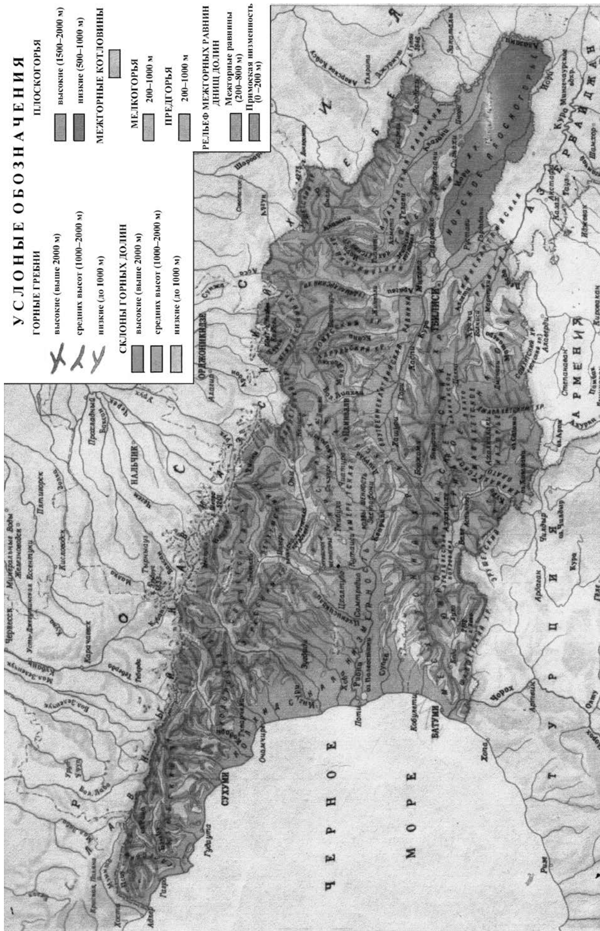
Рис. 3.1. Морфологическая карта Грузии
