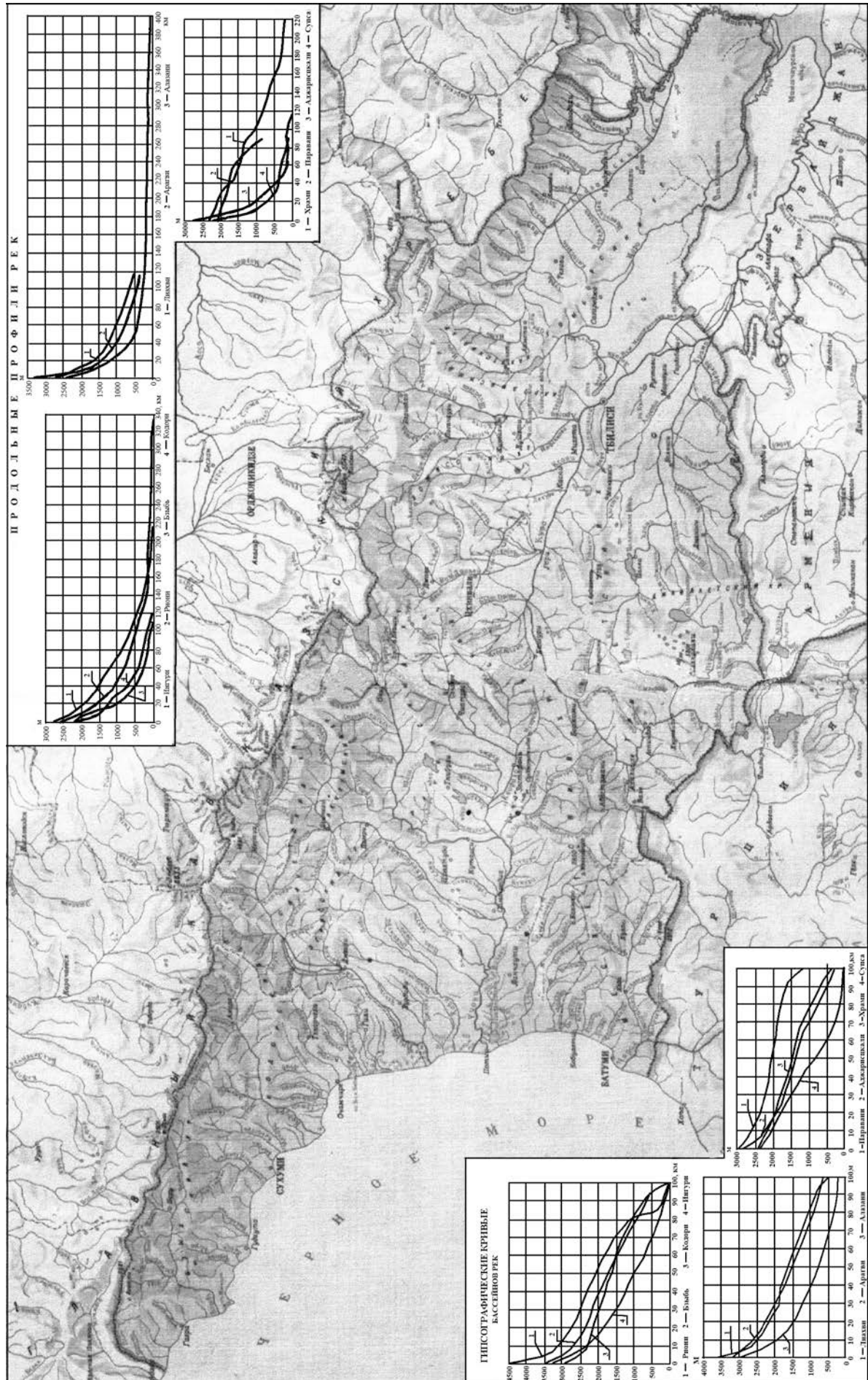
Рис. 3.4. Гидрографическая карта Грузии
