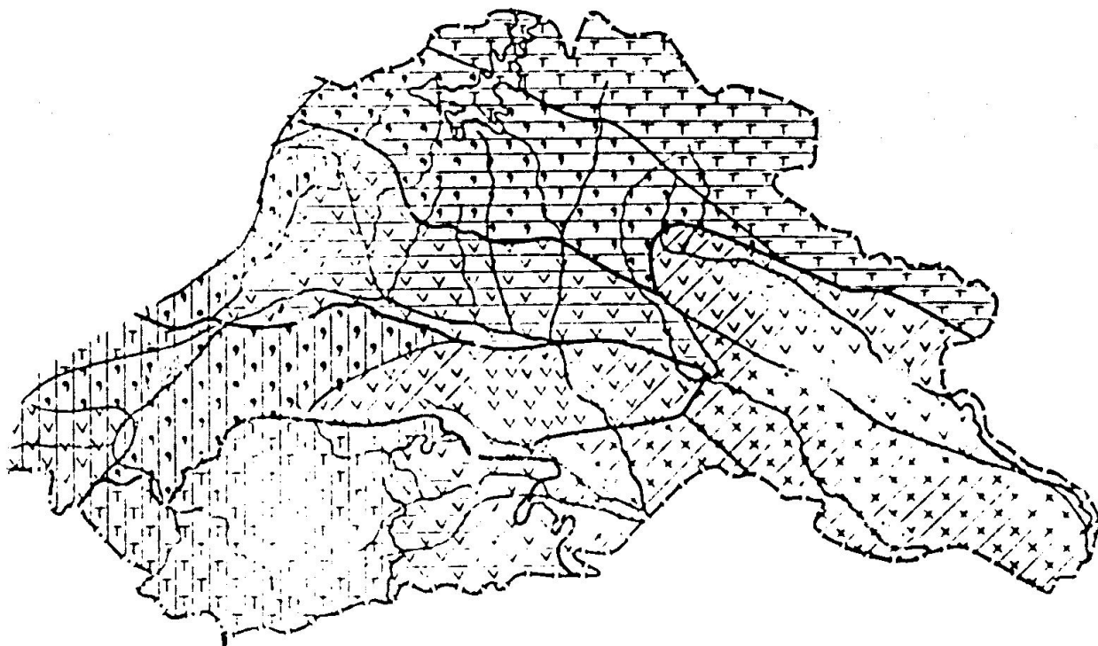
Рис. 4.2.60. Гидрохимический состав подземных вод Восточной Грузии.
