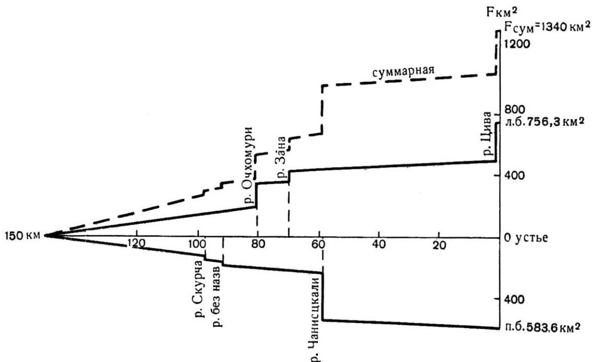
Рис. 4.1.30. График увеличения площади бассейна р. Хоби
