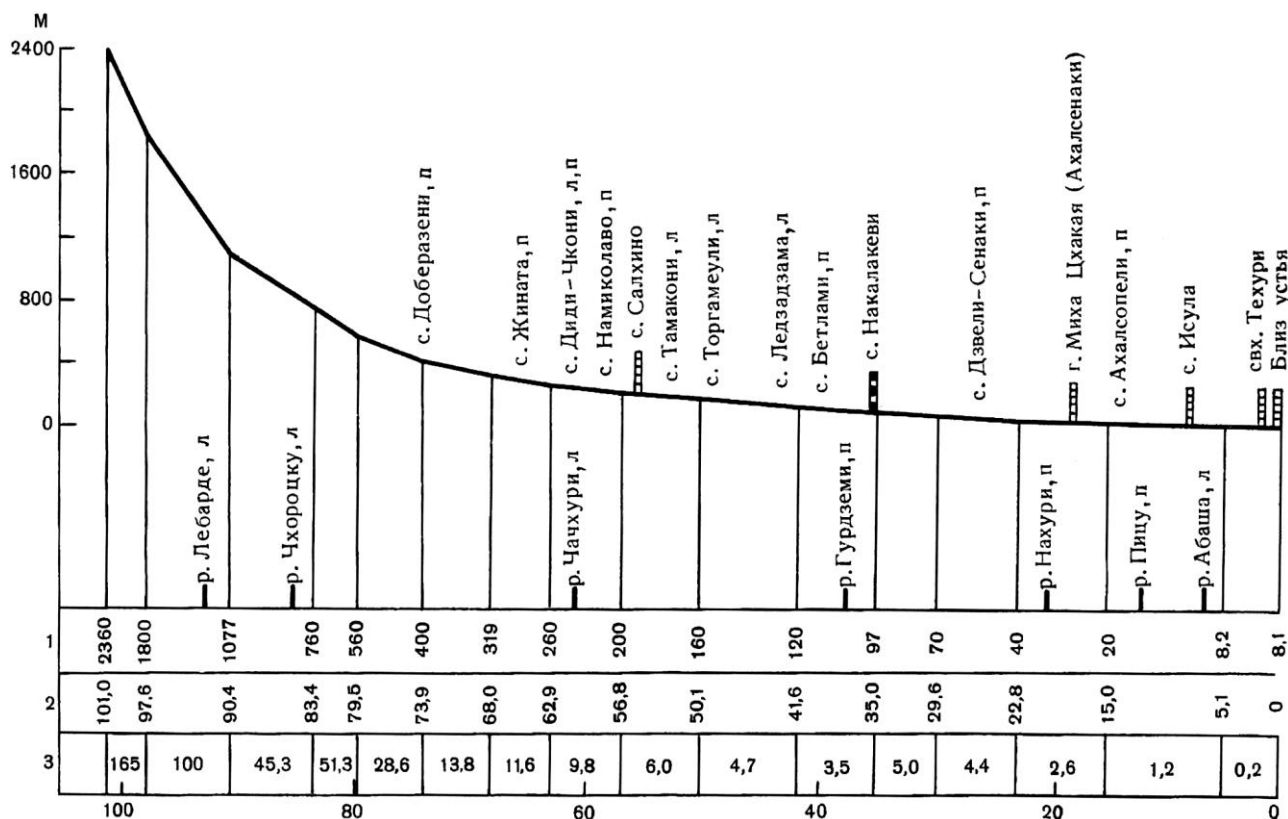
Рис. 4.1.41. Схематический продольный профиль р. Техура
