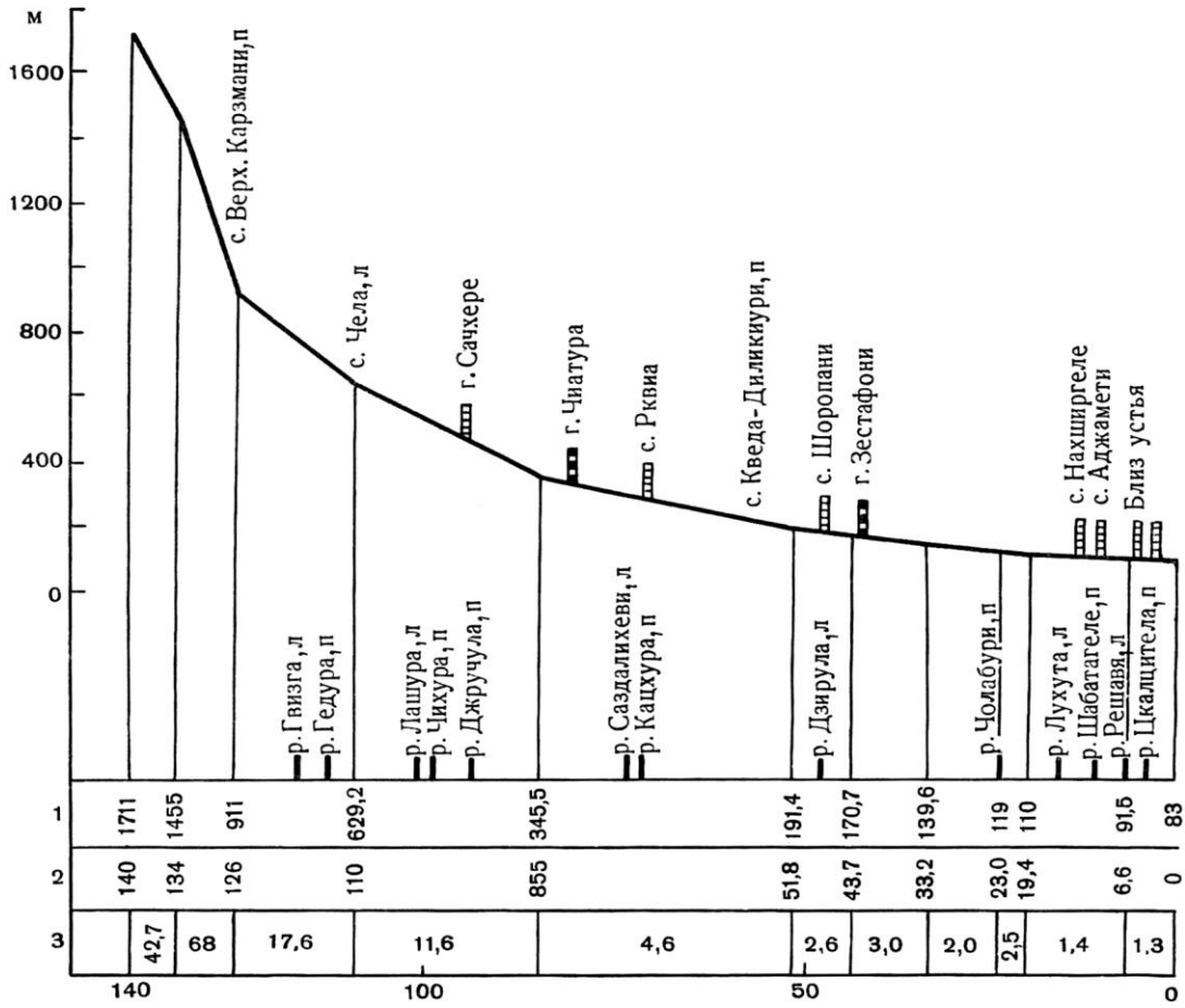
Рис. 4.1.35. Схематический продольный профиль р. Квирила
