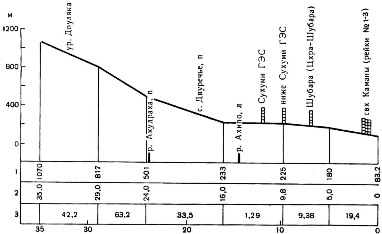
Рис. 4.1.15. Продольный профиль р. Западной Гумисты
