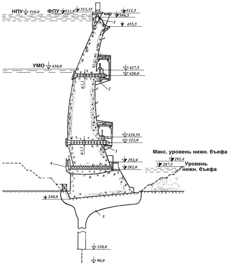
Рис. 4.2.48. Головной узел Ингурского (Джварского) водохранилища: а) план; б) поперечный профиль бетонной плотины
