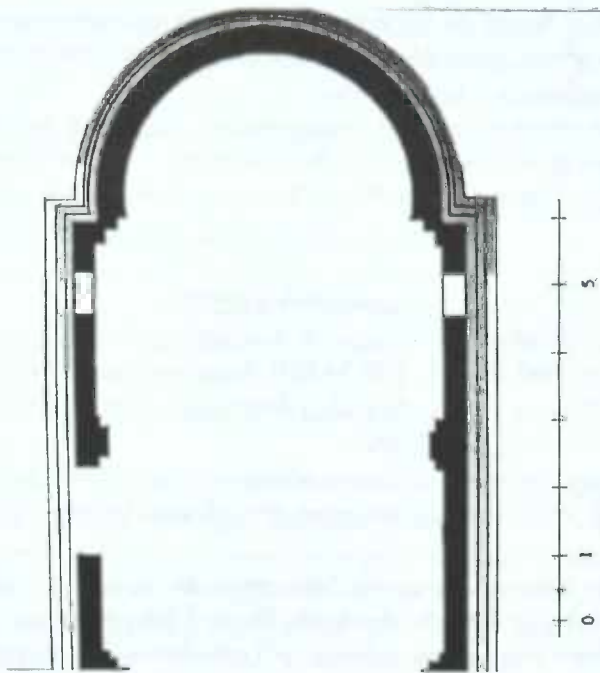
პირონიის ეკლესიის სქემატური გეგმა. შეასრულა გ. ყიფიანმა
